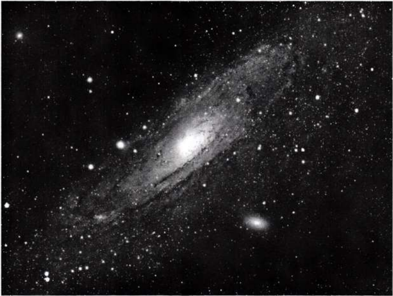
Рис. 7. Галактика
