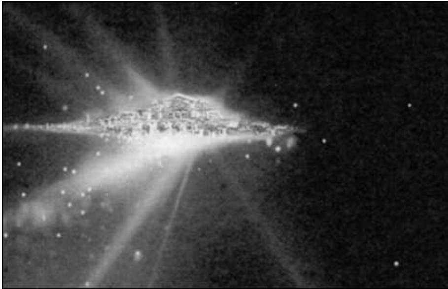
Город-рай. Фото телескопа НАСА «Хаббл» 26.12.1994 г.
