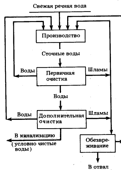
Р и с. 13. Схема очистки сточных вод на предприятии, сбрасывающем их в природные водоемы
