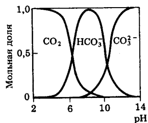
Р и с. 7. Влияние pH на состояние углекислого газа, растворенного в воде
