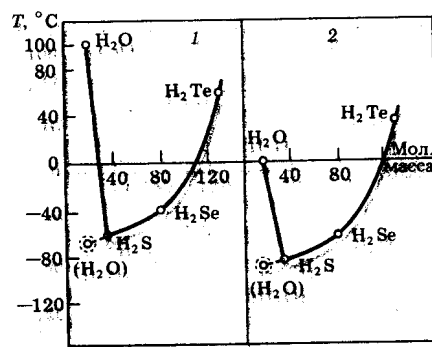
Р и с. 4. Температура кипения (1) и плавления (2) в ряду H_2O - H_2S - H_2Se - H_2Te . Пунктиром обозначены "нормальные" температуры кипения и плавления воды
