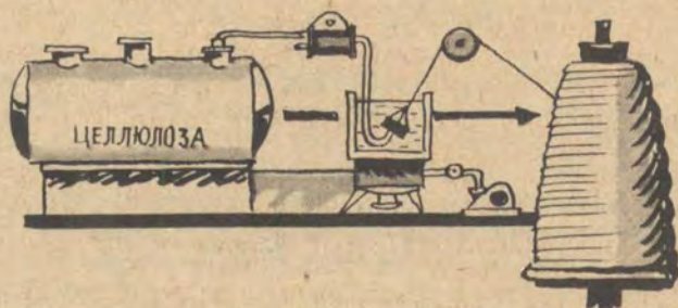
Схема получения вискозы.
