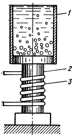
Рис. 5. Схема для кавитационной обработки деталей.
