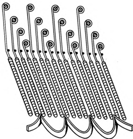
Схема 18. Заглушение обвитых струн полоской войлока
