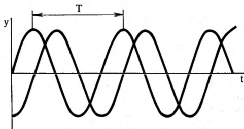
Схема 4. Сдвиг фаз колебаний
