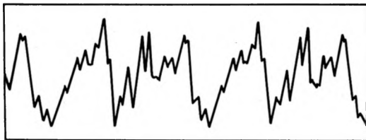
Схема 8. Форма колебаний скрипичной струны
