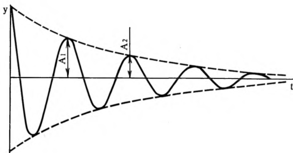
Схема 10. Затухающие колебания
