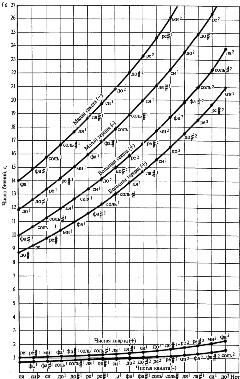
Схема 14. График биений интервалов настройки
