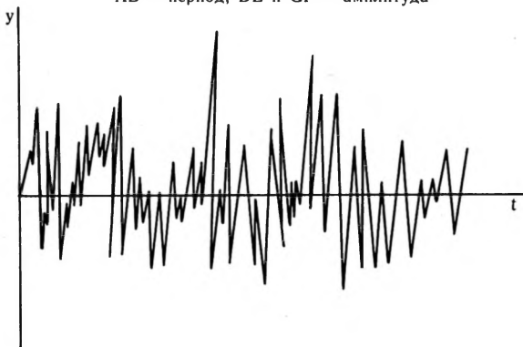
Схема 2. Белый шум
