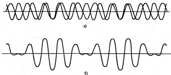
Схема 7. Сложение гармонических колебаний с небольшим различием частот
