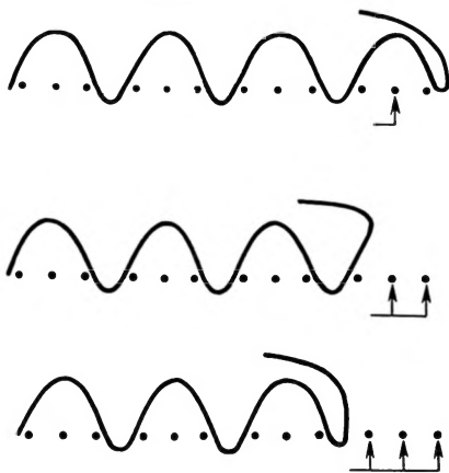
Схема 17. Заглушение гладких струн полоской войлока
