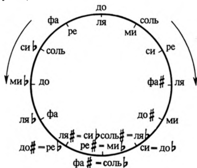
Схема 13. Квинто-квартовый круг гамм
