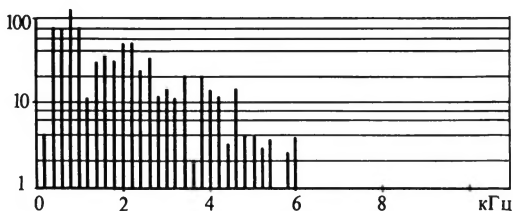
Схема 9. Спектр звука соль скрипки
