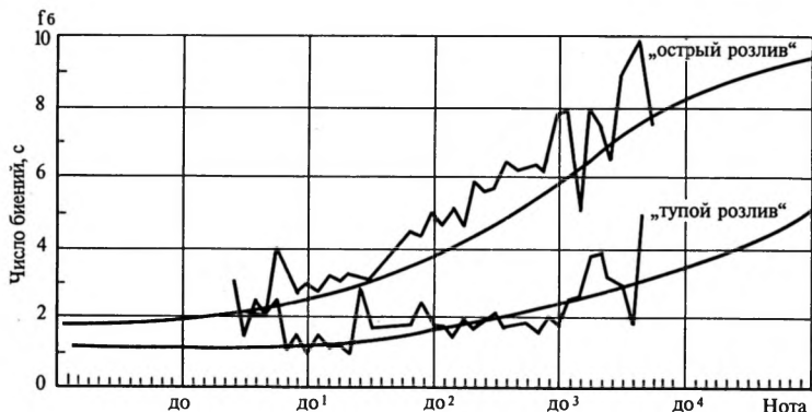
Схема 16. Законы «разлива» для язычкового инструмента
