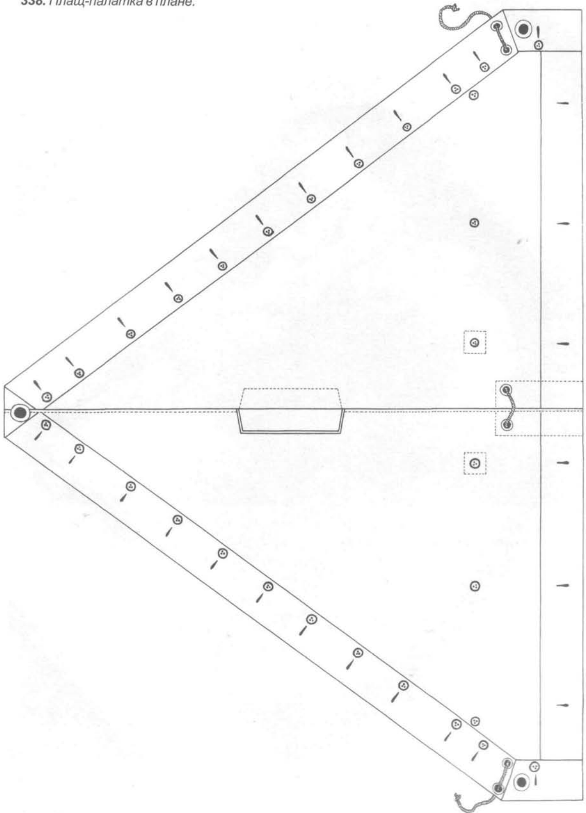
338. Плащ-палатка в плане.
