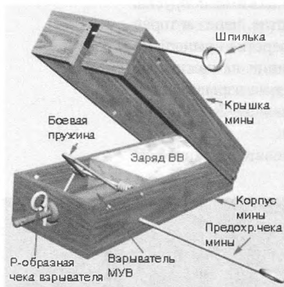
Мина-ловушка МС-2
