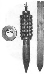
Противопехотная осколочная мина ПОМЗ-2
