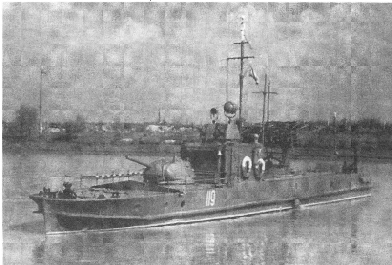
Бронекатер проекта 1124
