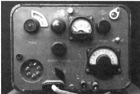
Радиостанция «Север»
