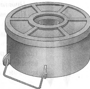
Противотанковая мина ТМ-41
