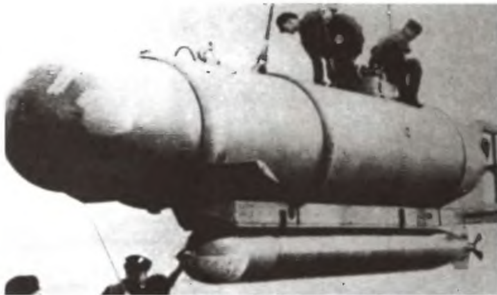
СМПЛ типа «Хехт» готовится к спуску на воду перед учебным выходом в море. Фото военного архива МО Германии
