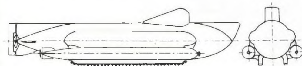
Проект «Специального корабля» — сверхмалой подлодки-амфибии, послужившей прототипом для «Морского дьявола»
