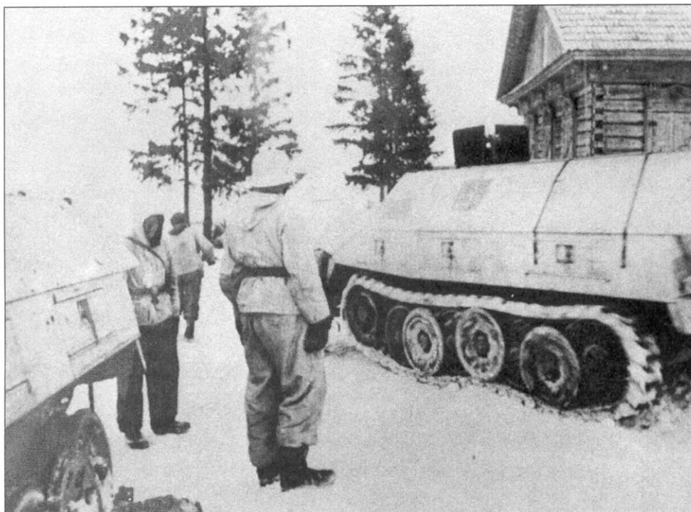
«Рабочая лошадка» гренедеров - бронетранспортер SdKfz 251/D. Модификация D была последним вариантом этой машины. В конструкцию было внесено большое количество упрощений для удешевления производства.
