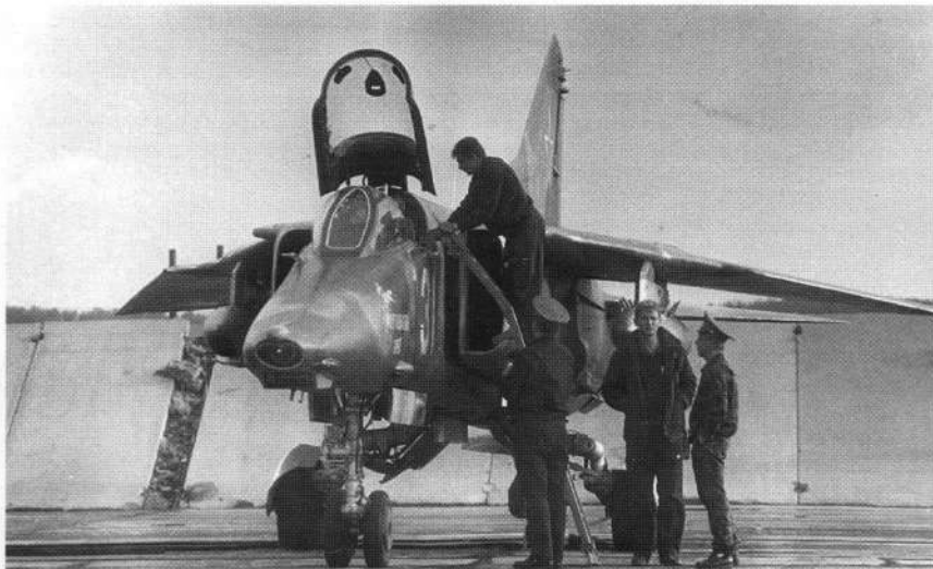
Технический экипаж выполняет послеполетное обслуживание МиГ-27К 266-й апиб. Аэродром Степь, лето 1990 г.
