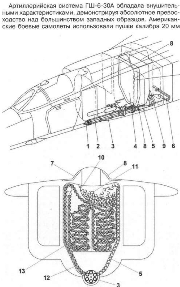
Стрельба из пушки ГШ-6-30А
