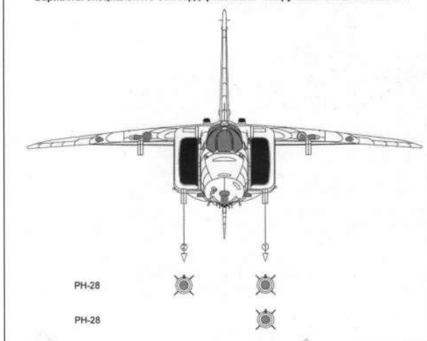
Варианты специального бомбардировочного вооружения самолета МиГ-27
