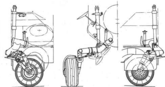
Основная стойка шасси самолета МиГ-27
