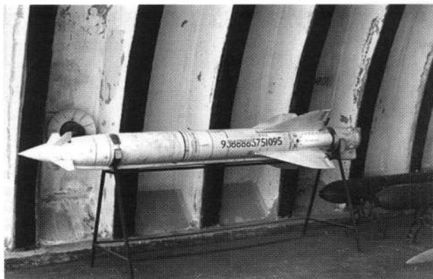
«Длинная рука» МиГ-27 – управляемая ракета X-23M (изделие 68M)
