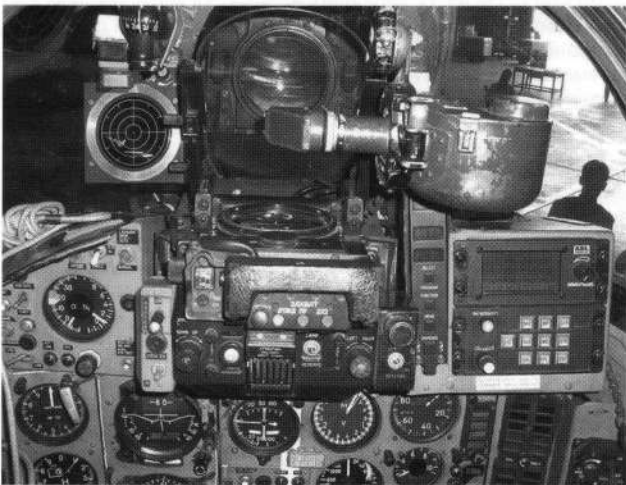
Кабина индийского МиГ-27М после модернизации
