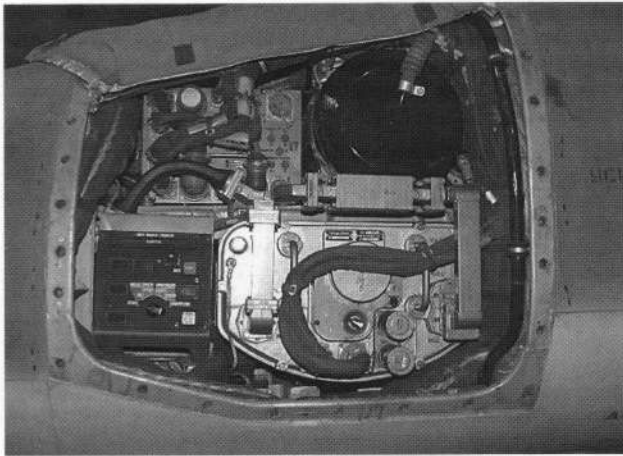
Бортовой пульт подготовки и контроля ППК (слева) и блоки помеховой станции СПС-141М «Сирень-ФШ» в отсеке носовой части МиГ-27К. Откинутый чехол сверху служит для защиты оборудования от осадков
