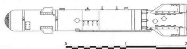
Корректируемая авиационная бомба КАБ-500Кр (изделие К07)
