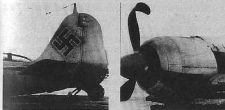
Последствия тарана (по немецкой терминологии — случайного столкновения) немецкого FВ-190 с советским истребителем
