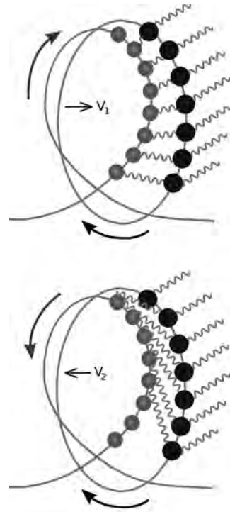
Рис.14. Схематическое изображение взаимодействия двух одинаково и
