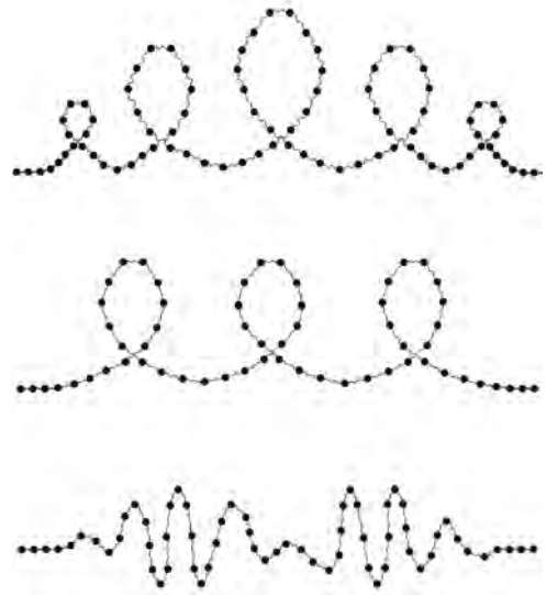
Рис.7. Элементарные частицы могут быть представлены сложными волнообразными возмущениями пространственной «решетки» (однако также не исключено, что основную их часть составляют возмущения «решетки» – хвостовые возмущения, – вызванные центральной конфигурацией).
