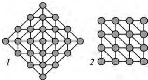
Рис.2. Различные представления плоского двумерного пространства (1 и 2); пространство 2 является однородным.
