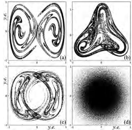
Рис.1. Странные аттракторы, сформированные дискретным по времени представлением траектории режима динамического хаоса в двух (а), трех (б) и четырех (с) потенциальных ямах (интервалы по времени равны периоду внешнего поля) – хорошо видна фрактальная структура аттракторов; квазислучайное – полученное на компьютере – распределение точек (д), представляющее шум с нулевым средним значением.
