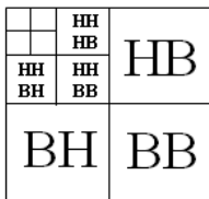
Рис. 6.6. Схема вейвлет-преобразования изображения: Н – фильтр низких частот, В – фильтр высоких частот
