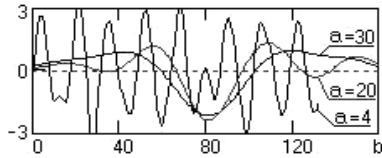
Рис. 2.30б. Фиксирование изменения фазы гармонического сигнала с изменением его фазы на 180^\circ в присутствии шумовых сигналов большой амплитуды
