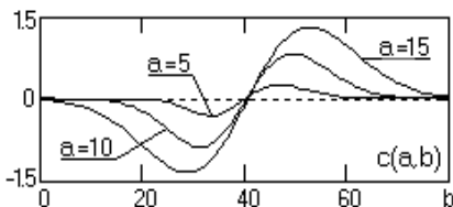
Рис. 2.28б. Вейвлет-анализ smoothed функции переключения
