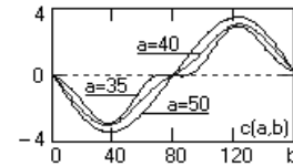
Рис. 2.31. Вейвлет-анализ суммы тренда ( y_1 ) и двух гармонических сигналов ( y_2 и y_3 )
