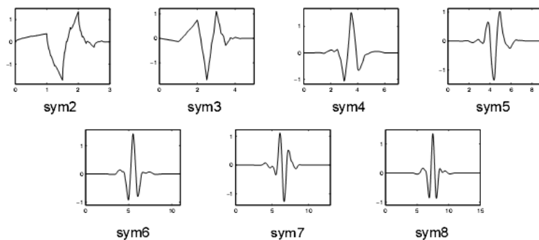
Рис. 5.10. Симплеты
