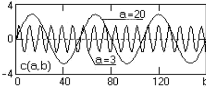
Рис. 2.29а. Вейвлет-анализ с помощью Мхат-преобразования различных колебательных функций: сумма двух гармоник
