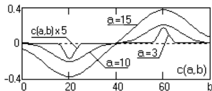
Рис. 2.28а. Вейвлет-анализ линейной функции переключения
