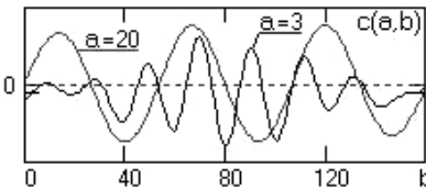
Рис. 2.29в. Вейвлет-анализ с помощью Мхат-преобразования различных колебательных функций: сумма двух гармоник, одна из которых модулирована по амплитуде функцией Гаусса
