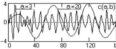
Рис. 2.29б. Вейвлет-анализ с помощью Мхат-преобразования различных колебательных функций: сумма двух гармоник, модулированных по амплитуде
