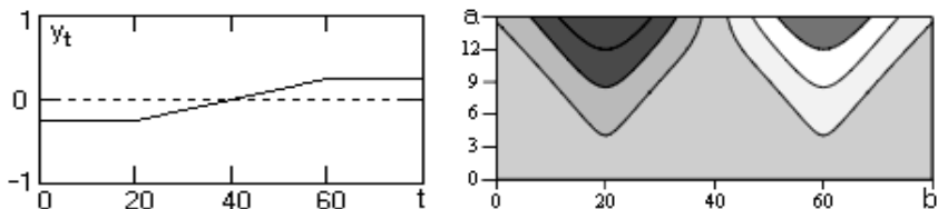
Рис. 2.28а. Вейвлет-анализ линейной функции переключения
