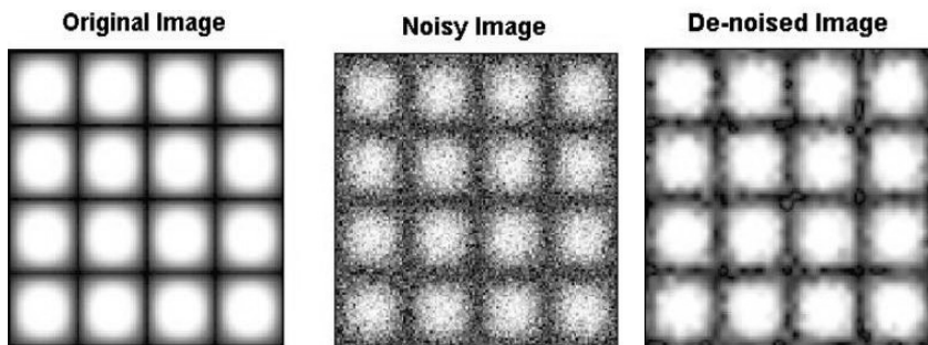
Рис. 1.8б. Масштабируемость алгоритма фильтрации шумов в двухмерном периодическом изображении. Слева – исходный и зашумлённый (в центре) рисунки; справа – рисунок с отфильтрованным шумом с помощью вейвлет-преобразования
