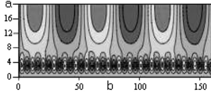
Рис. 2.29а. Вейвлет-анализ с помощью Мхат-преобразования различных колебательных функций: сумма двух гармоник
