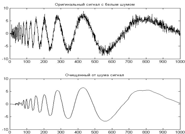
Рис. 1.7. Пример использования вейвлет-преобразования к зашумлённому квазигармоническому сигналу (с сильно меняющейся во времени амплитудой – в разы, и частотой – на порядки). Вверху – сигнал с шумом, достигающим вблизи минимума сигнала до 50 % его уровня, внизу – отфильтрованный сигнал с помощью вейвлет-преобразования
