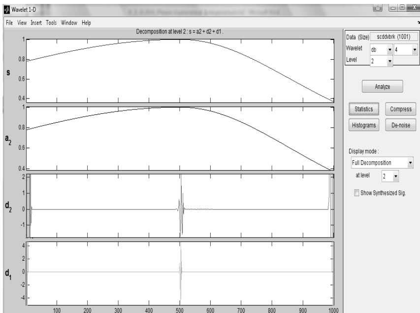
Рис. 5.36. Вейвлет-составляющие сигнала при использовании db4
