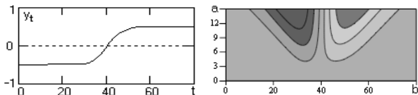
Рис. 2.28б. Вейвлет-анализ smoothed функции переключения
