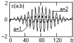
Рис. 2.31. Вейвлет-анализ суммы тренда ( y_1 ) и двух гармонических сигналов ( y_2 и y_3 )
