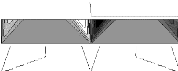
Рис. 2.21. Вейвлет-анализ конечного ступенчатого сигнала
