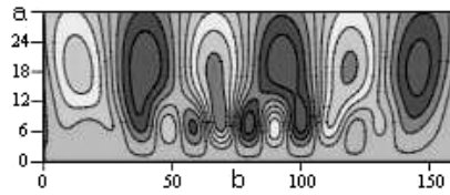
Рис. 2.29в. Вейвлет-анализ с помощью Мхат-преобразования различных колебательных функций: сумма двух гармоник, одна из которых модулирована по амплитуде функцией Гаусса
