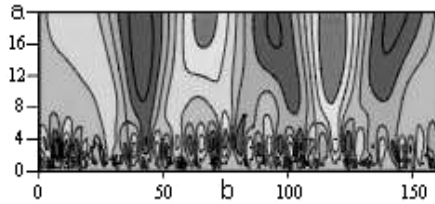
Рис. 2.29б. Вейвлет-анализ с помощью Мхат-преобразования различных колебательных функций: сумма двух гармоник, модулированных по амплитуде
