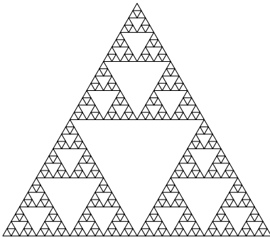
Рис. 1.7. Приближение \mathcal{S}'_6
