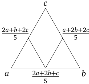
Рис. 3.1. Правило 1 : 2 : 2
