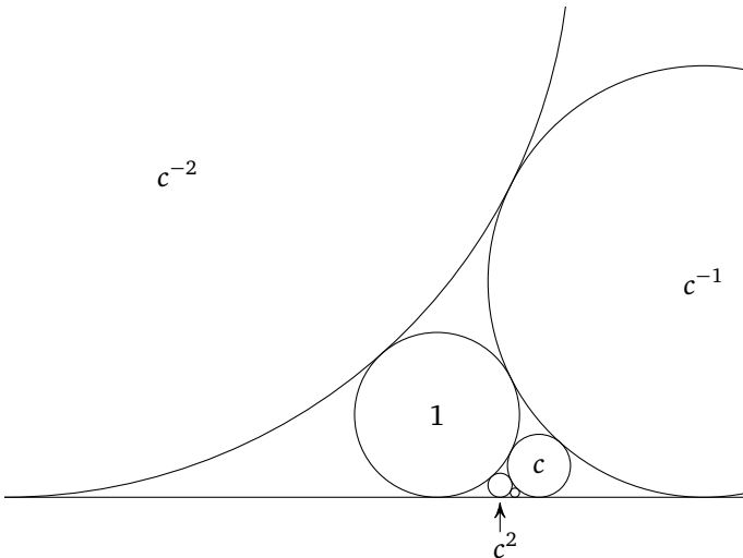
Рис. 5.6. Ковер \mathcal{A}_1
