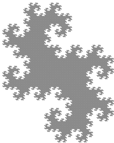
Рис. 3.8. Множество \mathcal{D}(S)
