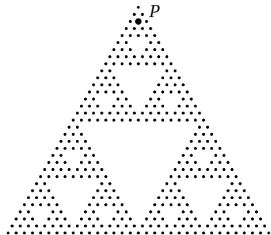
Рис. 1.8. Приближение \mathcal{S}_6
