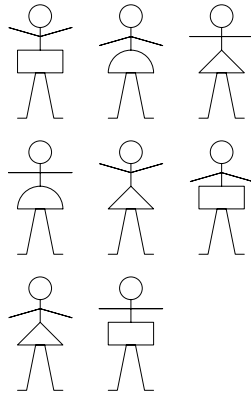
Рис. 2.21. «Пляшущие человечки». Добавить недостающего.
