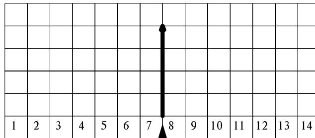
Рис. 10.2. Считается сумма очков, выпавшая на двух костях, и соответствующая фишка продвигается на одну клетку вперед. Мы в эту игру уже играли с мальчиками: суммы 1, 13, 14 вообще невозможны, наиболее вероятная сумма — 7.
