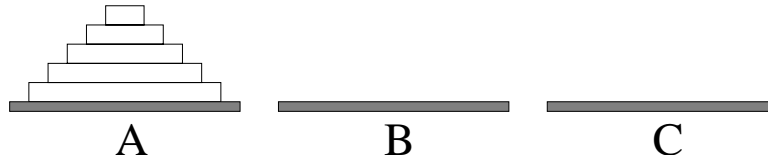
Рис. 2.6. Ханойская башня в начальной позиции.
