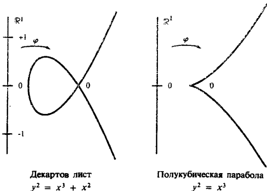
Параметризованные кубические кривые
