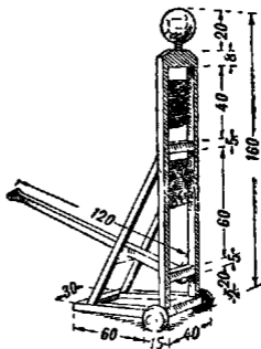
Рис. 101. Учебно-тренировочное чучело (с указанием размеров в сантиметрах).
