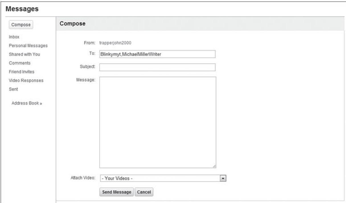
Рис. 17.5. Подготовка сообщения
