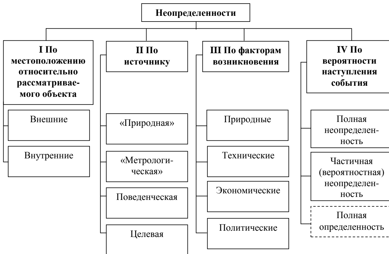
Рисунок 7 – Классификация неопределенностей
