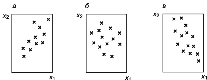
Рис. 5.7. Диаграммы рассеяния
