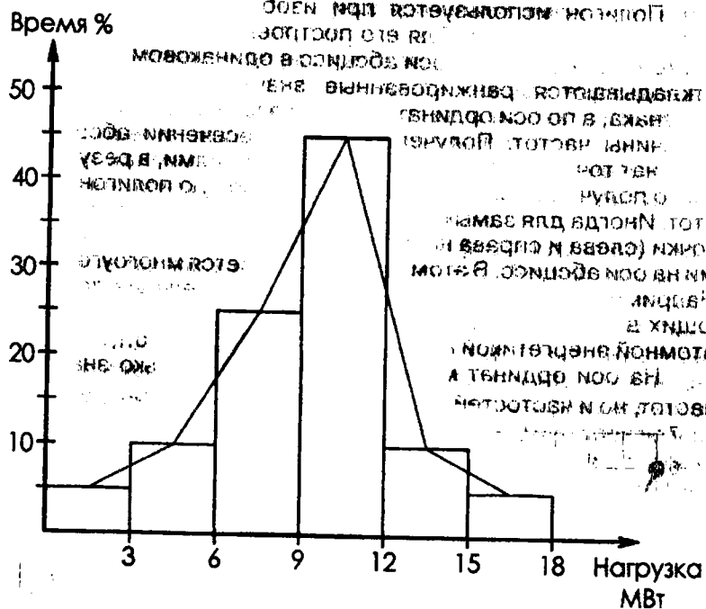
Рис. 6.2. Гистограмма электрической нагрузки промышленного предприятия (цифры условные)
