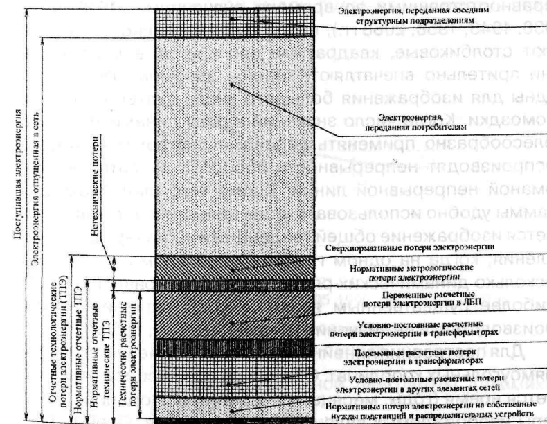
Рис. 4.7. Составные части структуры баланса электроэнергии
