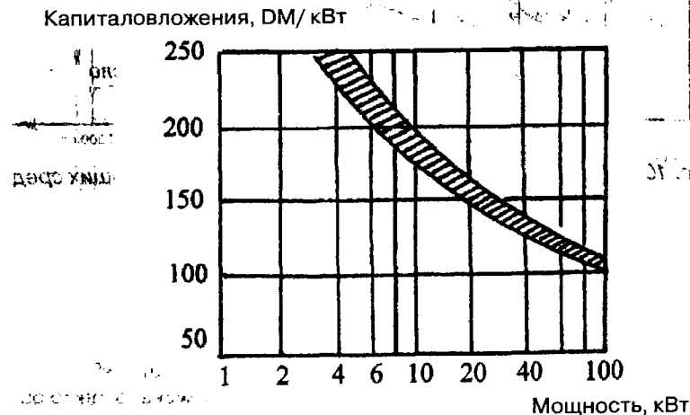
Рис. 10.7. Удельные капиталовложения в котеленую, работающую на газе или жидком топливе (1989 г.) (диаграмма с логарифмической шкалой) [14, с. 14, рис. 1]
