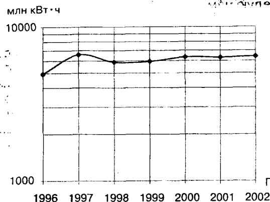
Рис. 5.5. Объемы выработки электроэнергии, млн кВт·ч, в Хмельницкой области за 1996–2002 гг.
