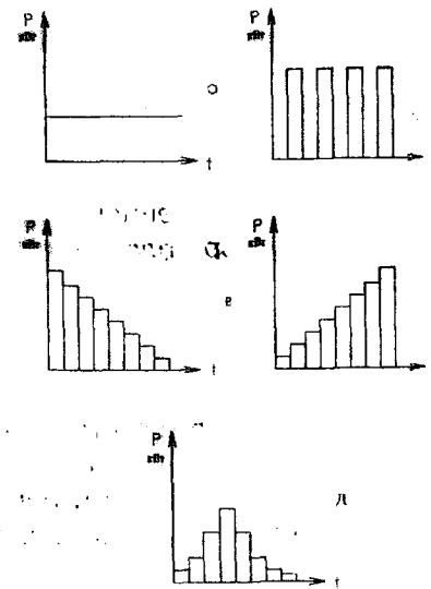
Рис. 6.6. Графики электрической нагрузки согласно рис. 6.5
