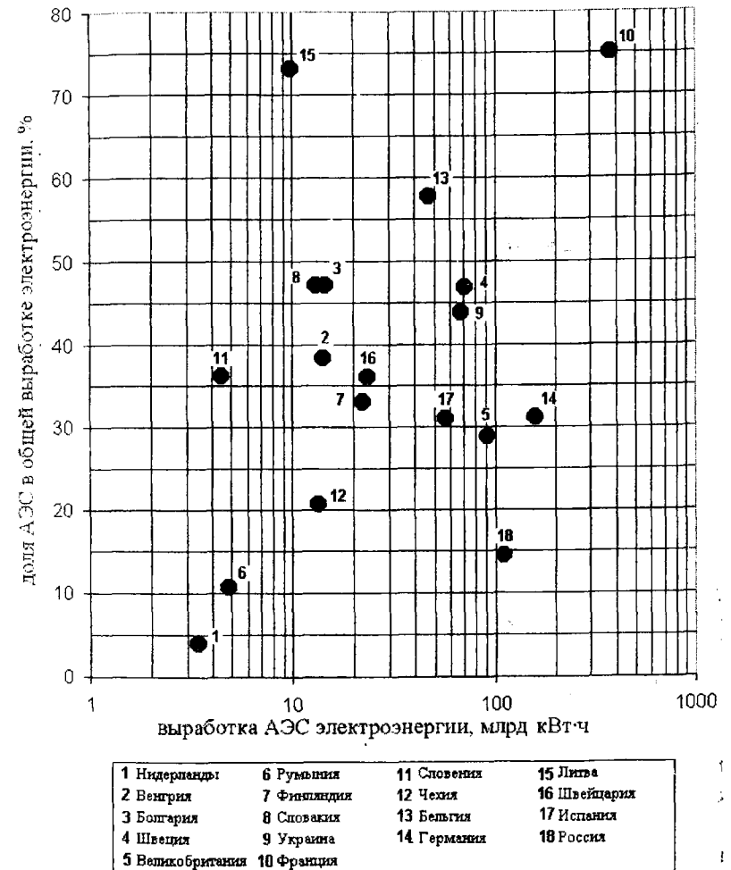
Рис. 3.12. Соотношение выработки электроэнергии действующими энергоблоками АЭС стран Европы в 1999 г. к проценту общего производства электроэнергии в стране
