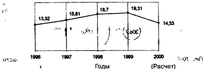
Рис. 10.2. Технологические потери электроэнергии при передаче в электрических сетях энергетических компаний Минэнерго Украины, %
