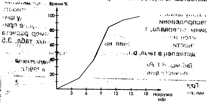
Рис. 6.3. Кумюлята распределения электрической нагрузки промышленного предприятия (цифры условные)
