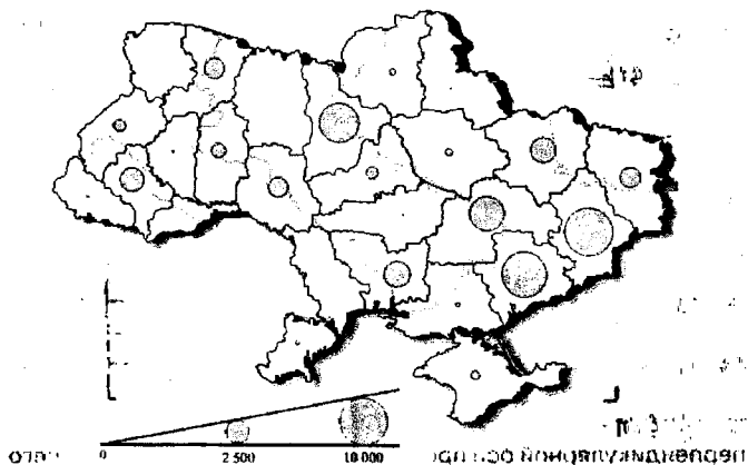
Рис. 7.5. Размещение генерирующих мощностей, МВт, по регионам Украины
