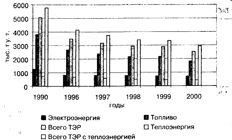
Рис. 3.4. Объемы потребления ТЭР по Хмельницкой области [11]
