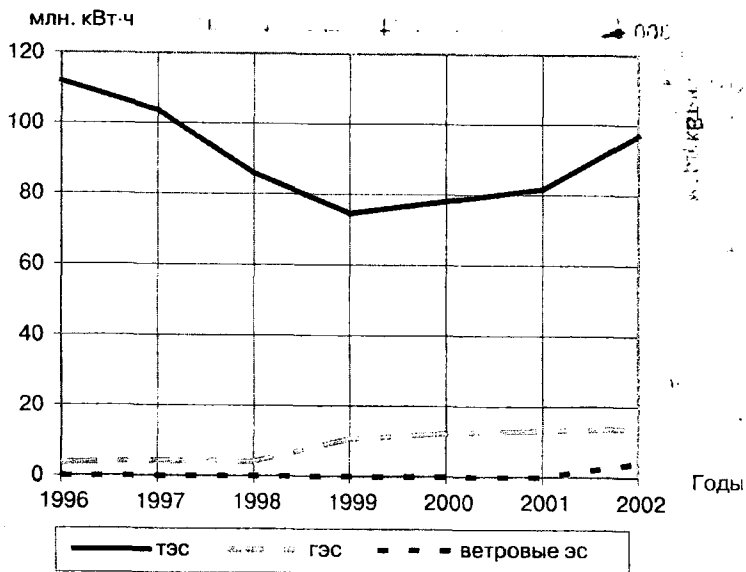
Рис. 5.3. Динамика производства электроэнергии, млн кВт·ч, в Хмельницкой области в 1996–2002 гг. по видам электростанций
