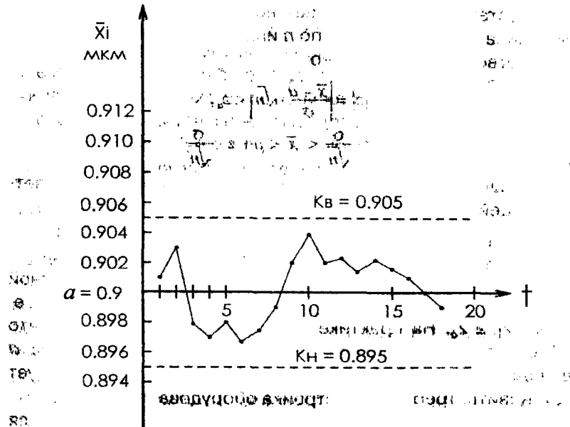
Рис. 8.1 Контрольная карта нанесения селективного покрытия энергосберегающего стекла (цифры условные)
