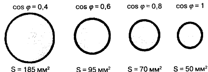
Рис.3.8. Диаграмма сечений жил трехфазной кабельной линии, передающей одинаковую активную мощность при разных \cos \varphi установок потребителей
