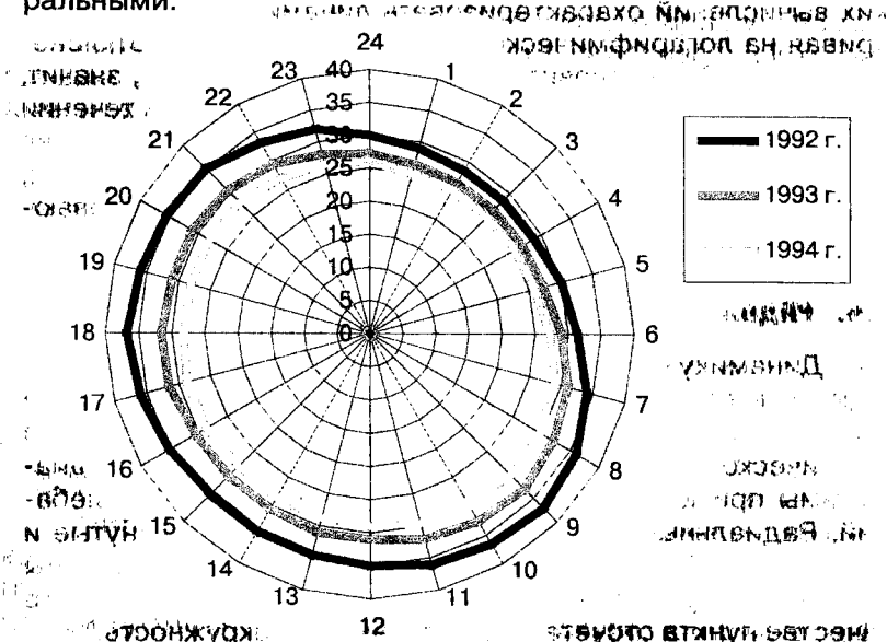
Рис. 5.6. Суточные зимние нагрузки энергосистемы Украины, МВт, в 1992-1994 гг.
