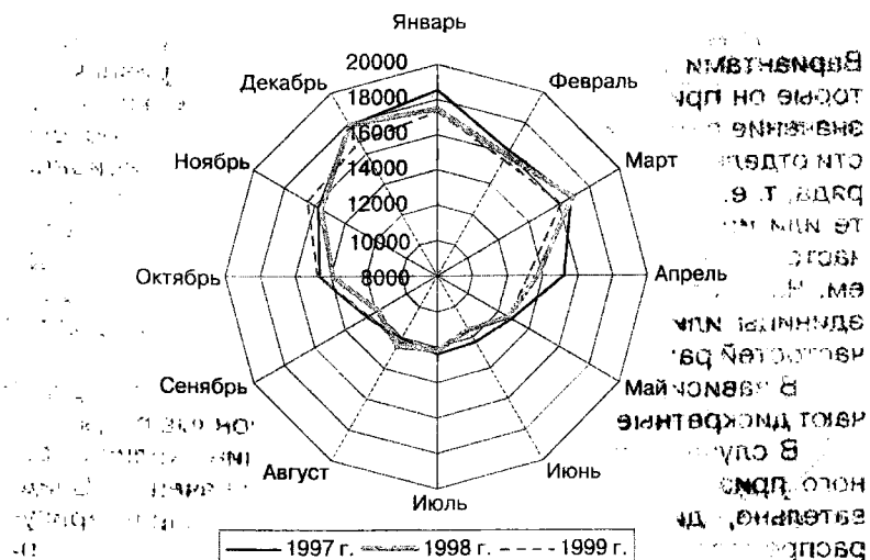
Рис. 5.7. Производство электроэнергии, млн кВт·ч, в Хмельницкой области в 1997-1999 гг.
