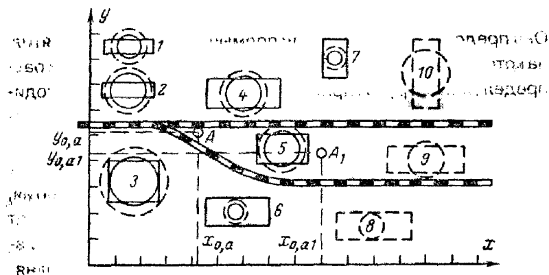
Рис. 7.6. Генеральный план промышленного предприятия с картодиаграммой и центром электрических нагрузок
