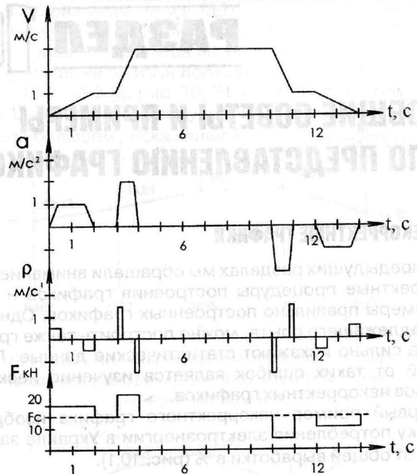
Рис. 9.2. Изменение параметров подъемной установки за цикл работы (цифры условные)
