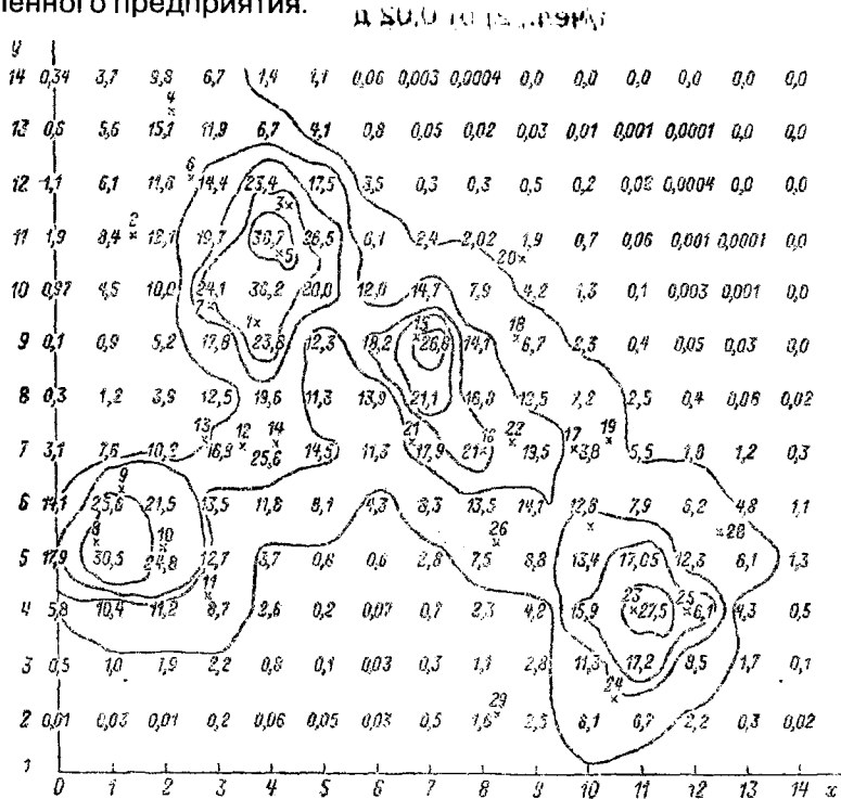
Рис. 7.2. Потенциальная функция нагрузок приемников электроэнергии промышленного предприятия
