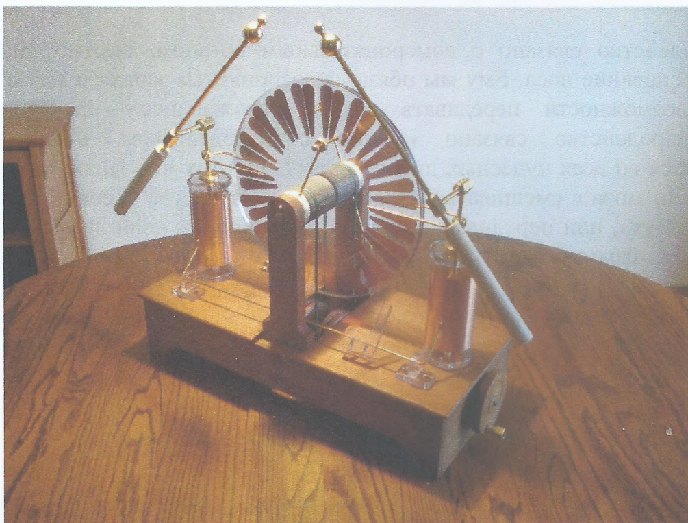
Рис. 12. Электрофорная машина
