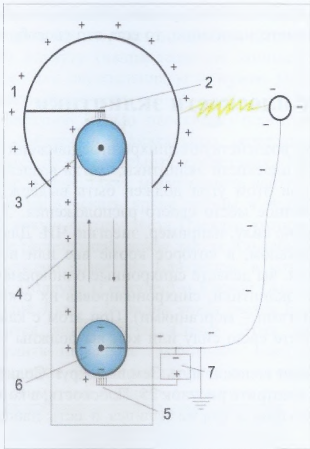
Рис. 13. Генератор Ван де Графа
