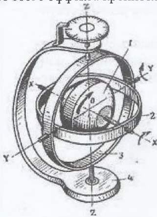
Рис. 1. Схема трехстепенного гироскопа:
