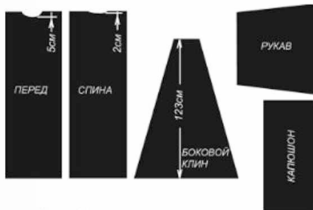
Рис. 3. Раскрой тау-мантии.
