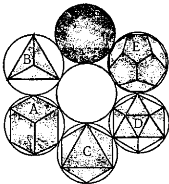
Платоновы тела, вписанные в сферу
