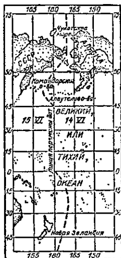
Линия перемены дат (часть линии)
