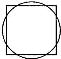
К задаче «Квадратура круга»
