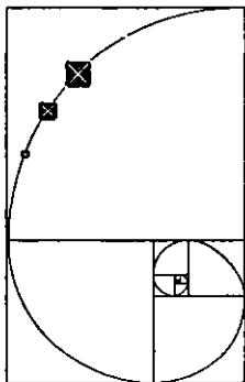
Логарифмическая спираль на плато в Гизе
