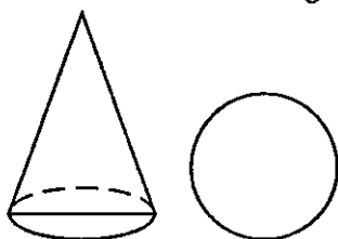
Конус: вид спереди и сверху
