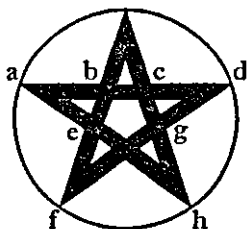
Божественная пропорция (золотое сечение) в пентаграмме
