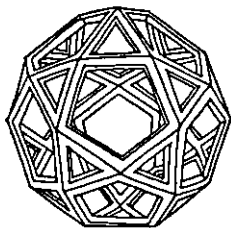
Многогранник Леонардо (иллюстрация к книге Луки Пачоли «De Divine Proportion» — «О Божественной пропорции»)
