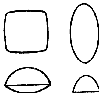
Кабошон
