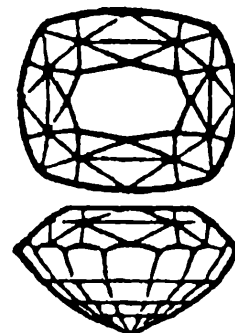
Цейлонская огранка
