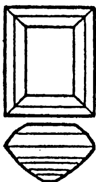
Ступенчатая огранка
