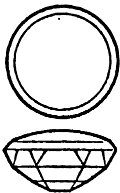
Смешанная огранка
