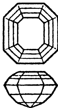
Изумрудная огранка
