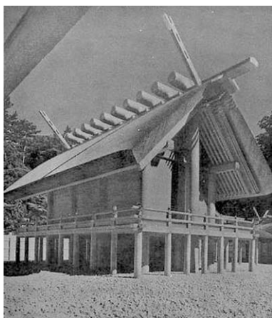
Рис. 55. Каркасный храм в городе Исэ
