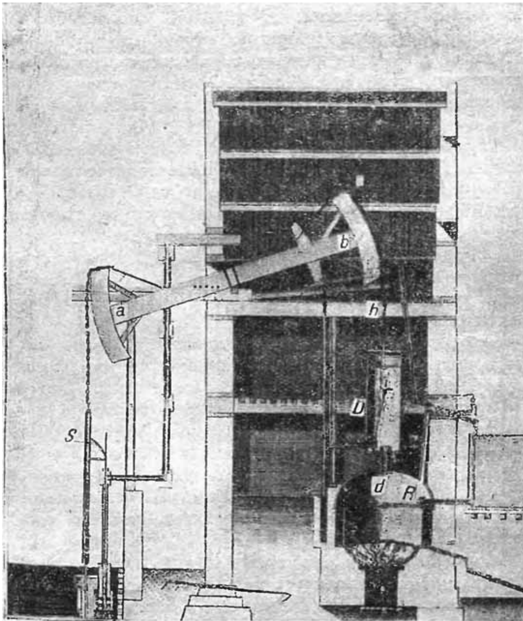
Машина Ньюкомэна.
