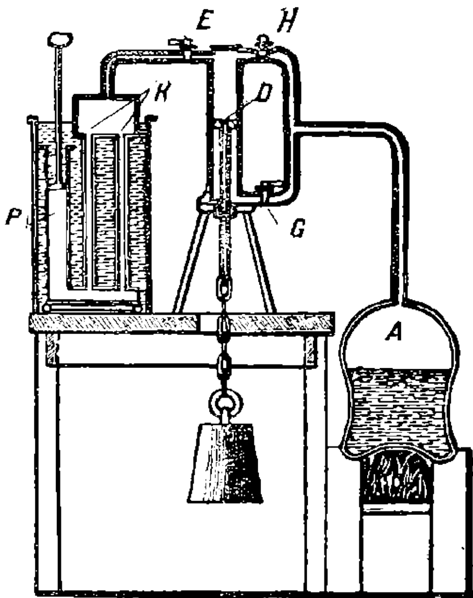
Схема действия первых уаттовских моделей с конденсатором. При небольшом подъеме поршня в насосе P пар из верхней части
