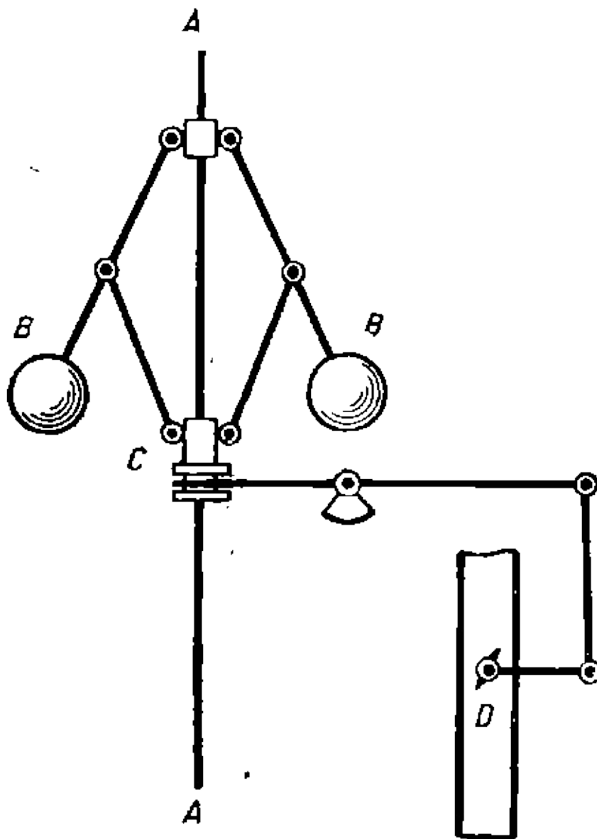
Центробежный регулятор.
