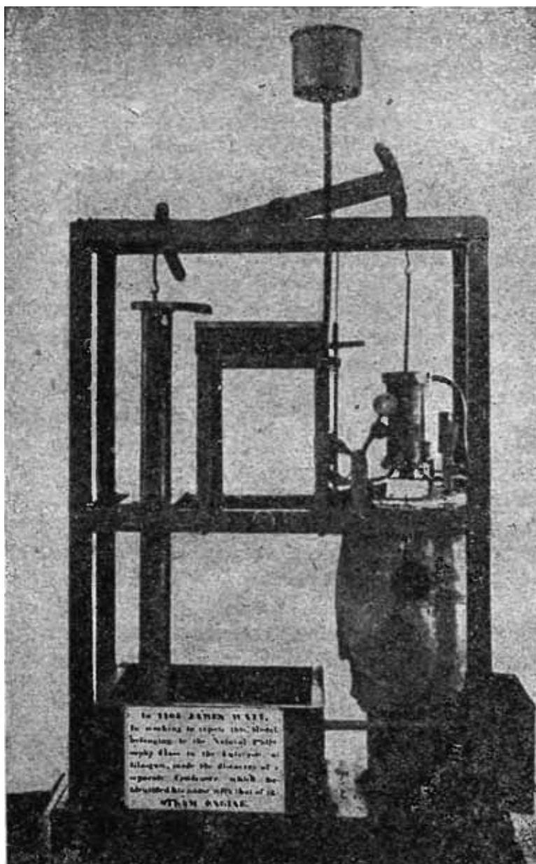
Модель машины Ньюкомэна, над которой работал Уатт.
