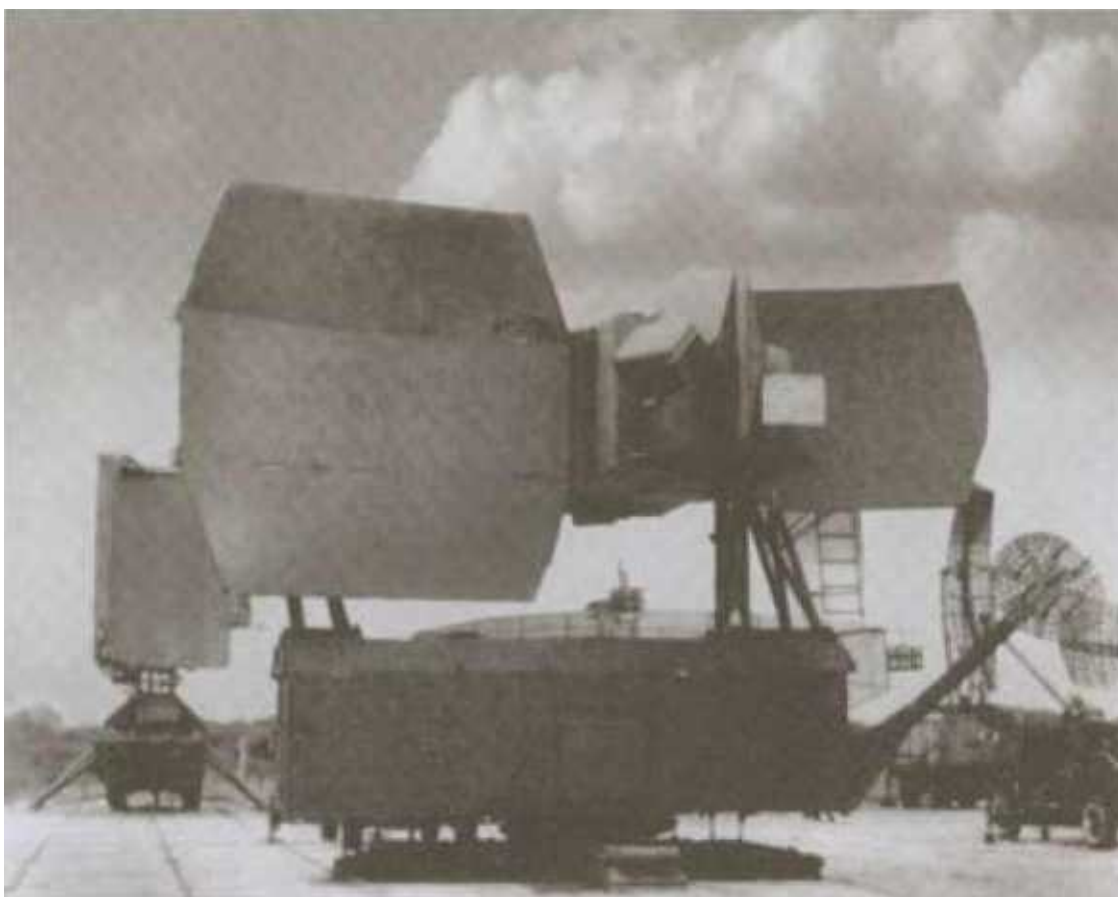
Антенный пост радиолокатора подсвета цели.
