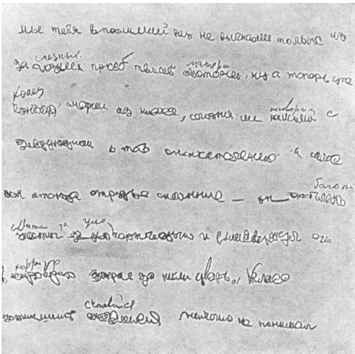
Страница рукописи Н. Островского, написанная при помощи самодельного транспаранта.
