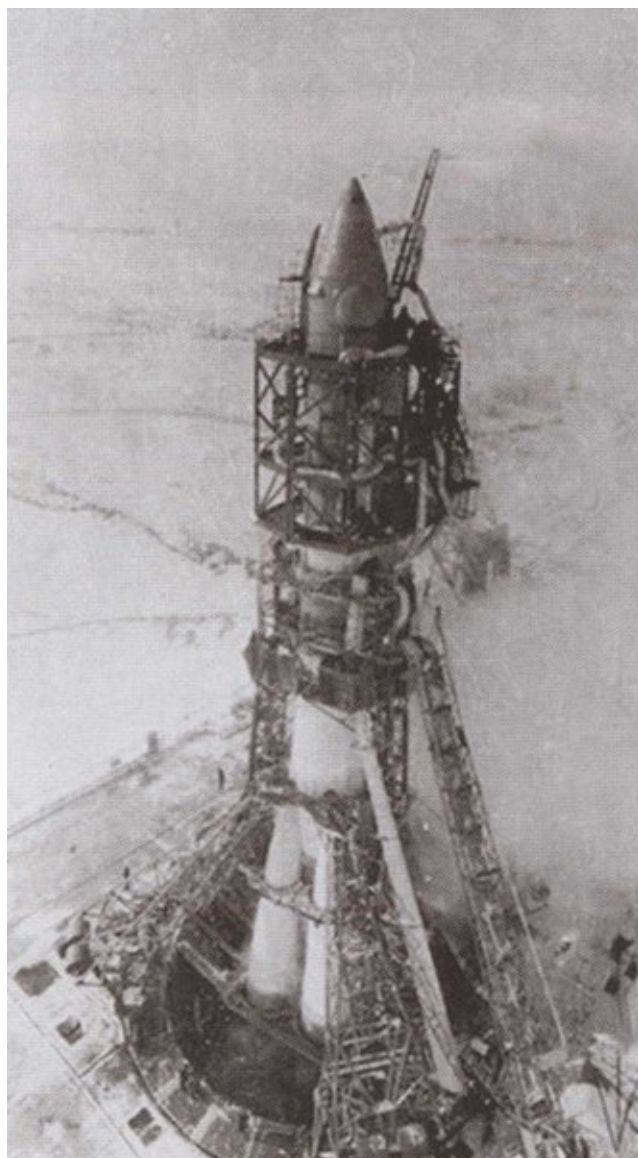
Стартовая площадка ракеты «Восток-1»
