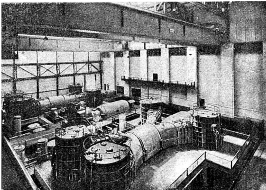
Величайшая в мире паротурбинная установка в Чикаго мощностью в 208 000 киловатт
