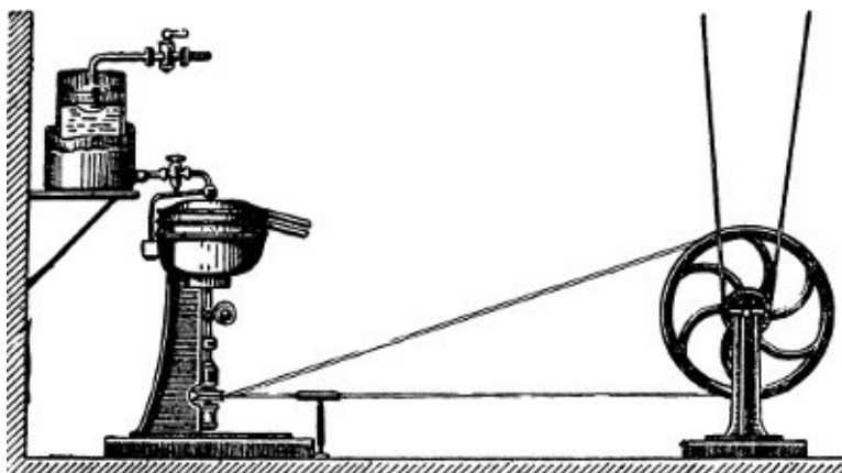
Передачи Лавалья для увеличения числа оборотов сепаратора
