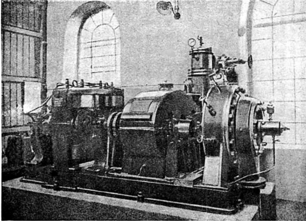
Турбина Лавая мощностью в 100 лош. сил, соединенная с динамо-машиной
