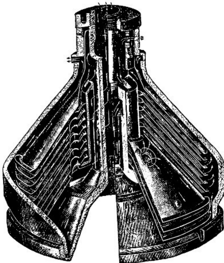
Разрез барабана сепаратора «Альфа — Лаваль»
