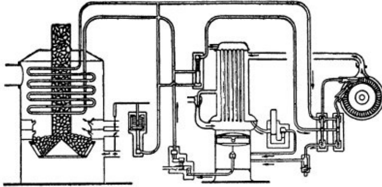
Разрез котла Лавалья
