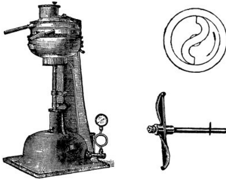
Турбинный сепаратор Лавалья и турбинное колесо
