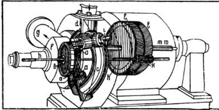
Турбина Лавалья со снятым кожухом
