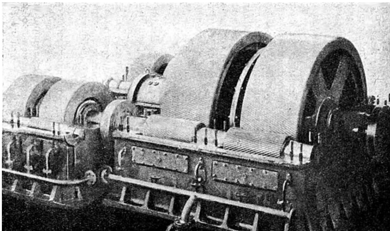
Современная геликоидальная передача Лавая для судовой турбины мощностью в 6 000 лощ. сил
