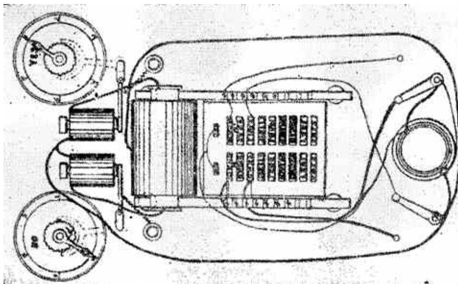
Генератор Эдисона с нижним расположением якоря.
