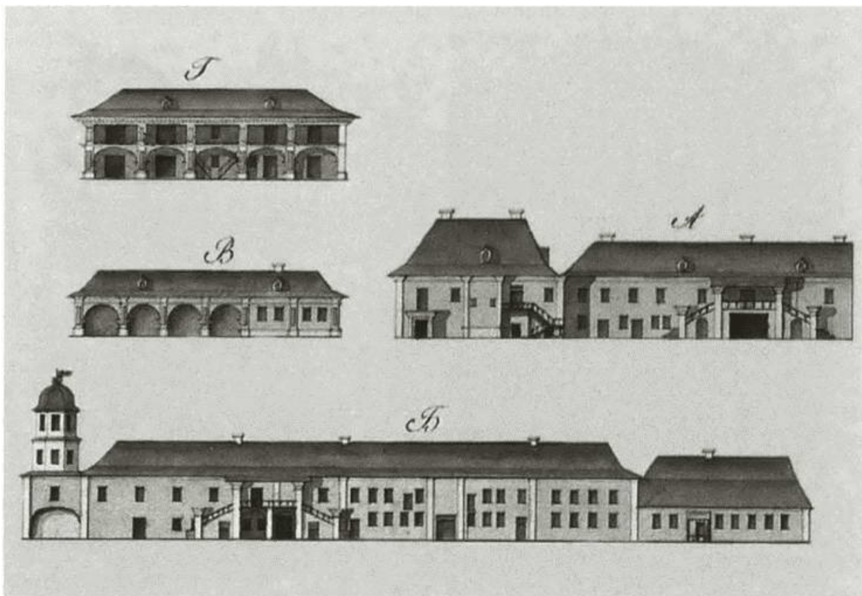
Ансамбль господских хором и конторы на Невьянском заводе: план (вверху) и дворовые фасады (внизу). Чертеж первой половины XIX в.
