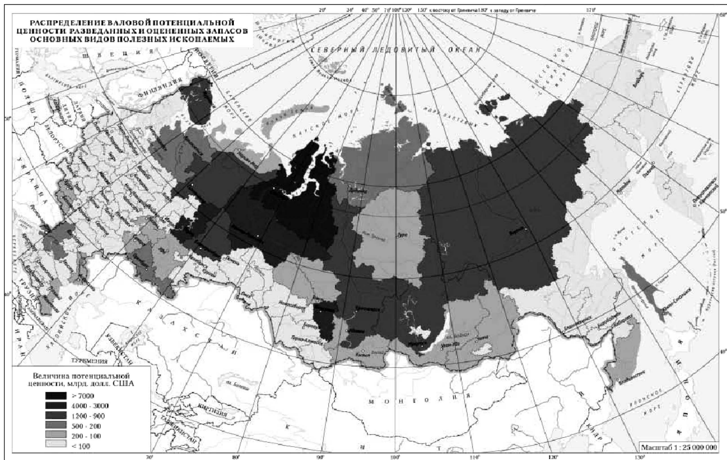
Рис. 1.2.10. Распределение валовой потенциальной ценности разведанных и оцененных запасов основных видов полезных ископаемых
