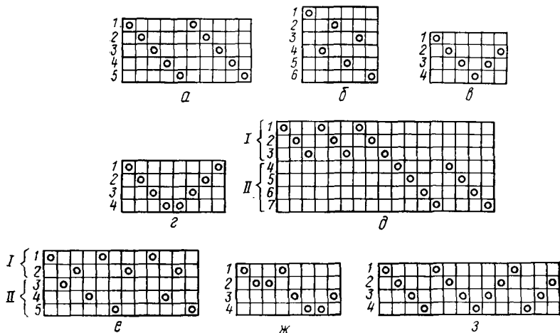
Рис. 5. Виды проборок
