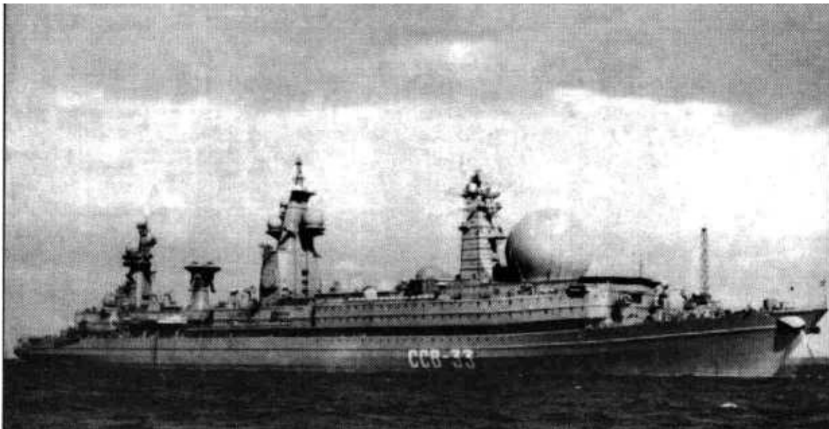
Корабль-атомоход радиоэлектронной разведки «Урал»
