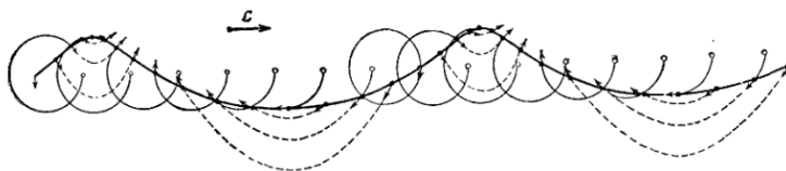
Рис. 437. Связь линий тока и круговых путей в бегущих водяных волнах. Горизонтальный ряд точек показывает частички поверхности воды в состоянии покоя, дуги окружностей — пути, проходимые ими по направлению часовой стрелки. Соединив маленькие острия стрелок , мы получаем профиль распространяющейся вправо волны в конце следующего промежутка времени. Круговые траектории вычерчены для каждой второй стрелки.
