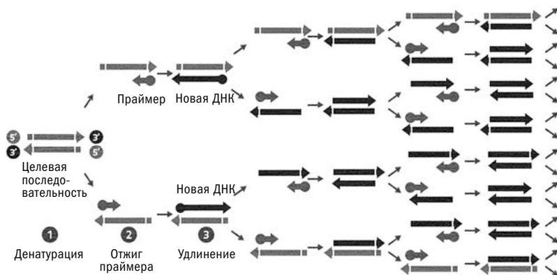
Рис. 17. Схема полимеразной цепной реакции (ПЦР)
