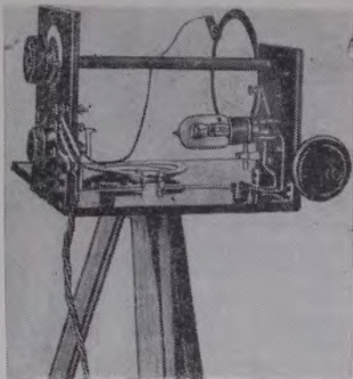
Рис. 13. Вид УКВ-радиопередатчика на длинну волны 2—4 м, работавшего снаружи камеры при ее испытании 30.XII 1926 г. в лаборатории В. Л. Дурова.
