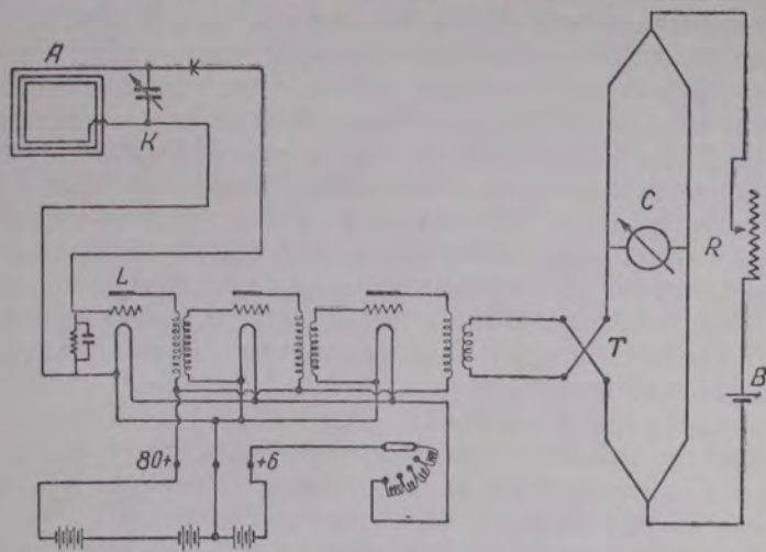
Рис. 10. Первоначальная схема «электромагнитного микроскопа» для приема и регистрирования биоэлектромагнитных волн при акте мышления.
