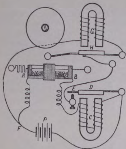
Рис. 1. Схема первого в мире радиоприемника, изобретенного А. С. Поповым и названного им «грозоотметчик».
