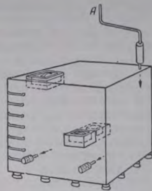
Рис. 18. Экранирующая камера итальянского ученого Ф. Кацамали:
