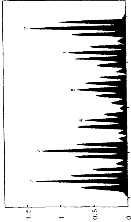
Рис. 2. Динамика отклонений орбитального углового момента Солнца от среднего значения в единицах стандартного отклонения, сглаженная по 3-летним интервалам за период 1800 - 2000 гг.
