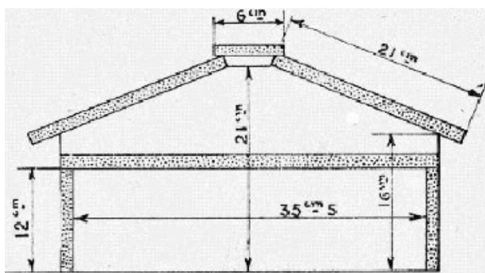
Поперечное сечение двухскатной крыши
