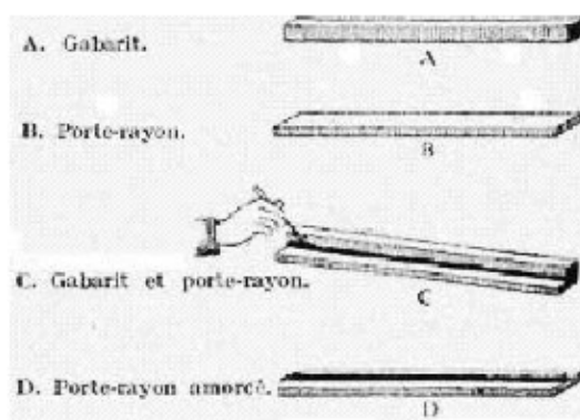
А. Шаблон для формирования полоски стартера на планке. В. Планка. С. Шаблон и планка. D. Планка с полоской стартера.
