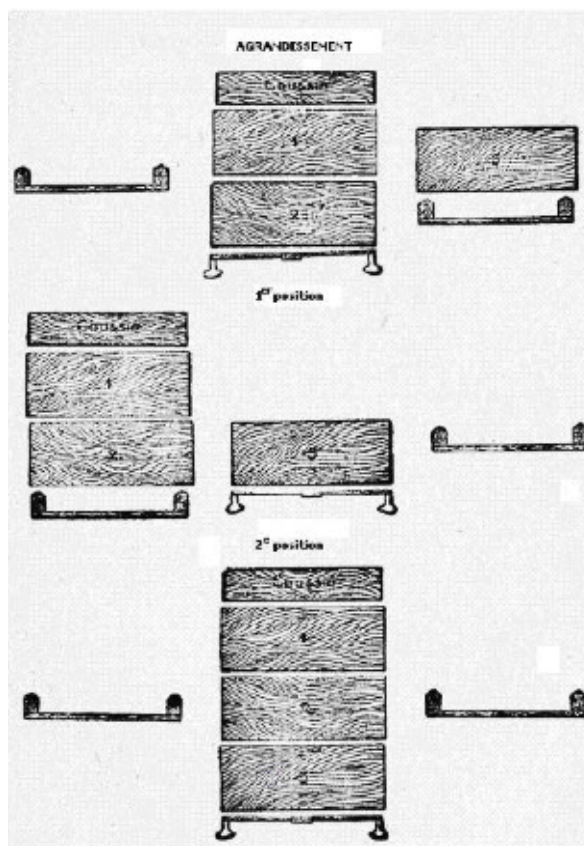
Расширение улья
