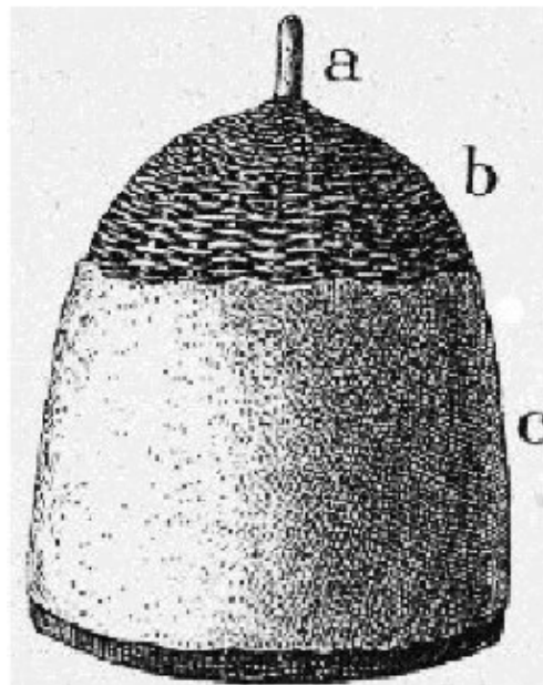
Skep плетеный из лозы: а-ручка; b-прутья лозы; c-покрытие (смесь глины и коровьего помета).
