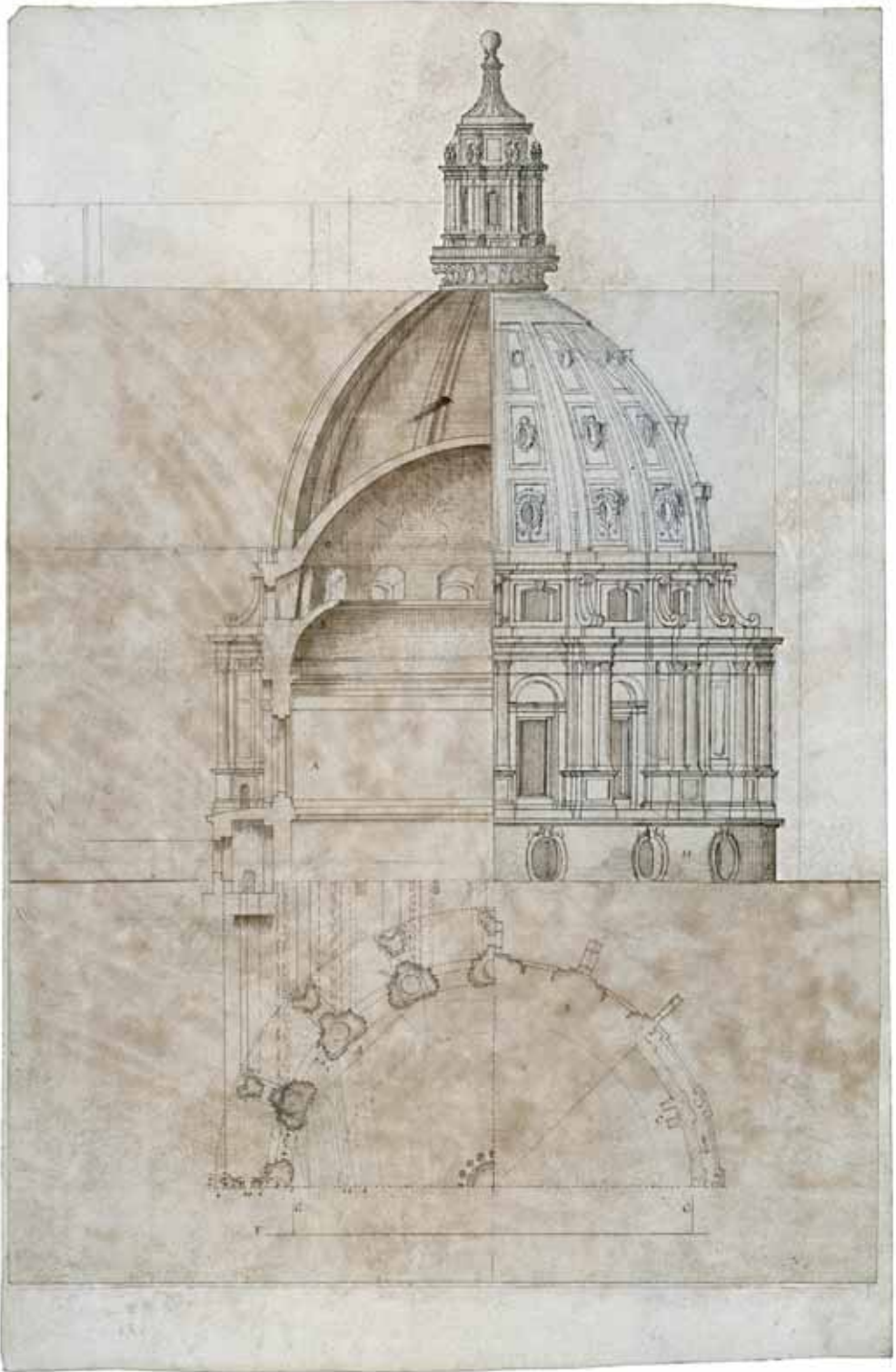
Архитектурный рисунок Микеланджело.
