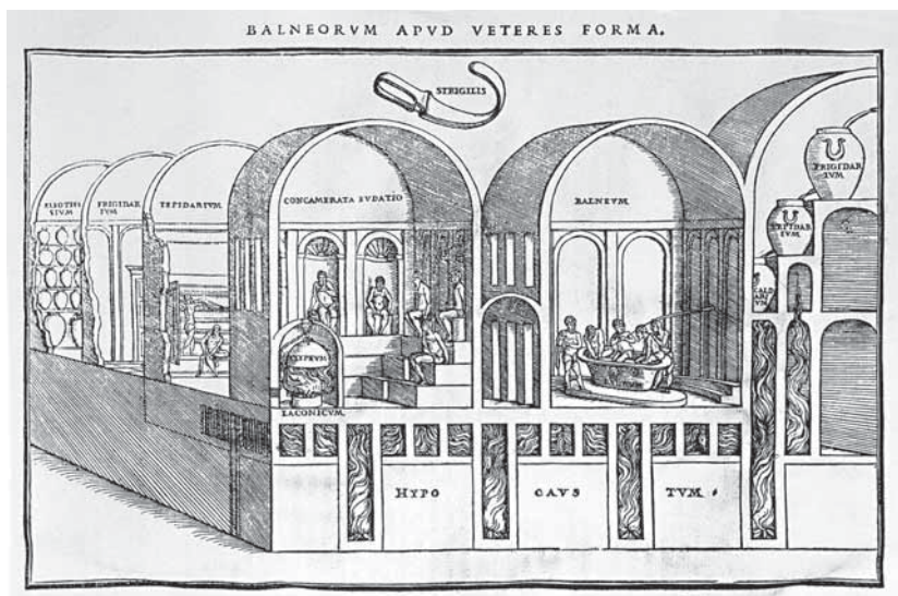
Римская баня с горячей, холодной и паровой баней и системой отопления комнат.
