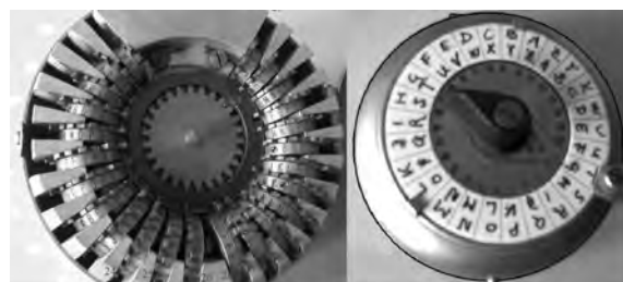
Рис. 17. Венгерская ручная шифрмашинка (вид снизу и сверху).
