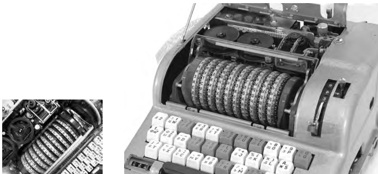
Рис. 1. Вид на роторы, клавиатуру и печатающий механизм «Фиалки»
