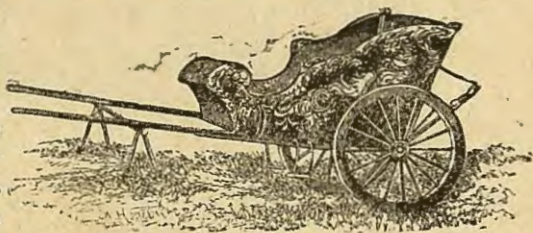
Одноколка Петра Великаго.
