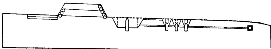
Разрез линии прусского ретраншемета под Кольбергом. (По чертежу русского инженера из корпуса Румянцева.)
