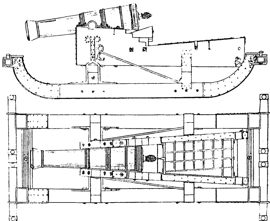
Пушка с лафетом на полозьях (для зимней кампании): сверху — вид сбоку; внизу — вид сверху. (ЦВИА, ВУА, № 17814.)
