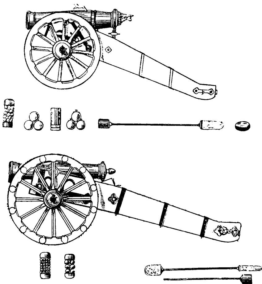
Вверху: единорог полупудовый. Внизу: гаубица шуваловская полупудовая. (ЦВИА, ВУА, № 17780 и 17788.)
