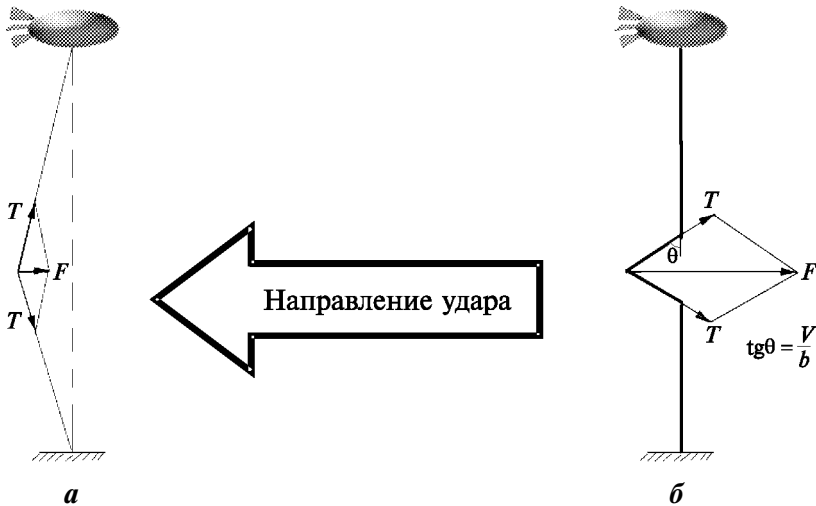
Схема сил, возникающих при квазистатическом а и динамическом б отклонении троса при ударе
