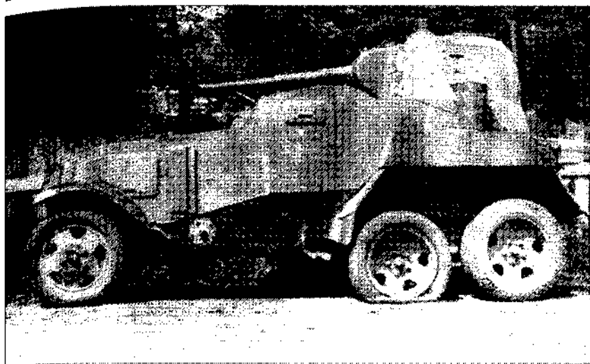
Трофейный советский броневлаutomобиль БА-10 со знаком РОНА
