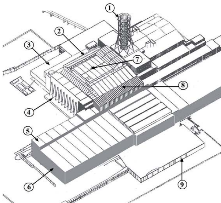
Рис. 5. Общий вид объекта «Укрытие». Обозначения: 1 – венттруба; 2 – северные щиты покрытия; 3 – каскадная стена, 4 – контрфорсная стена, 5 – деаэрационная этажерка; 6 – машинный зал, 7 – кровля, покрывающая центральный зал, 8 – южные щиты покрытия; 9 – южная пионерная стена
