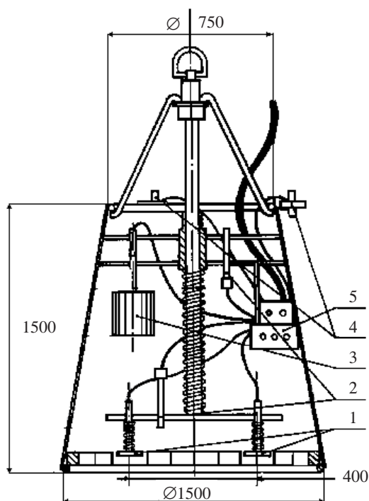
Рис. 17. Детекторы, находящиеся внутри буя. Обозначения на схеме (размеры в мм): 1. Датчики плотности теплового потока. 2. Термометры. 3. Детекторы мощности дозы гамма-излучения. 4. Анемометры. 5. Панели коммуникаций
