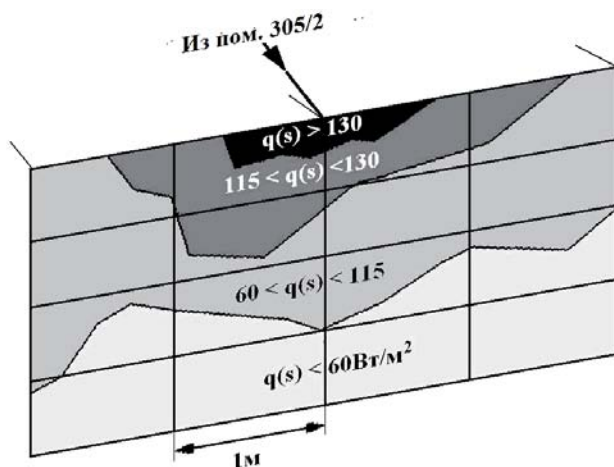
Рис. 19. Распределение плотности тепловых потоков на западной стене пом. 213/2
