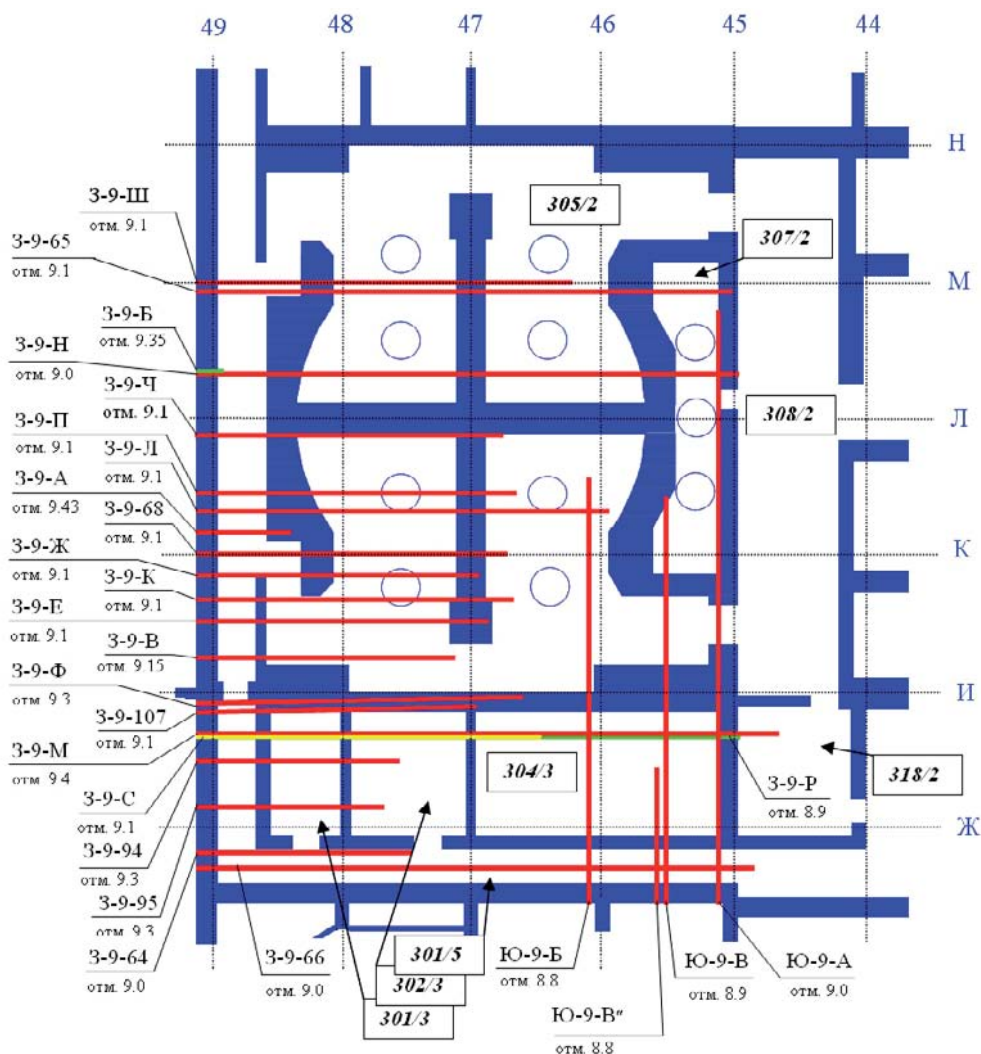
Рис. 2. Схема скважин, пробуренных в 4-ом блоке на отметках +8.800 \div +9.400 м ([3], [6]). Наклонные скважины: 3-9-Ф (горизонтальный угол -1^\circ ) и 3-9-107 (горизонтальный угол -1^\circ , вертикальный -1^\circ )
