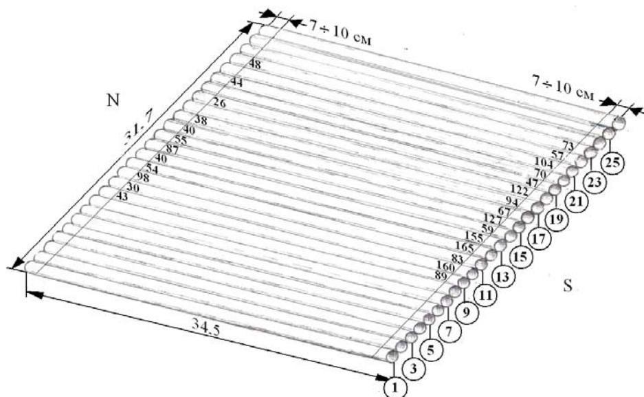
Рис. 25. Результаты измерения доз с помощью накопителей ДПГ-03 на трубном настиле, Р/ч. Выполнены 12.10.86 г. Данные в пределах погрешности измерений ( \pm 30\% ) совпадают с данными, полученными 03.10.86 и 24.10.86.
