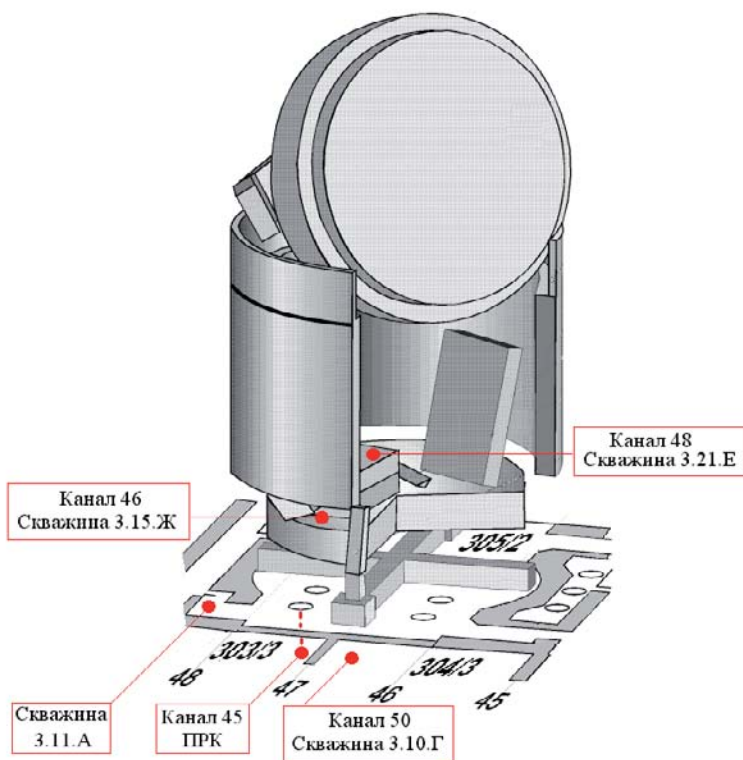
Рис. 3. Схема расположения нейтронных каналов системы «Финиш» летом 1990 г.
