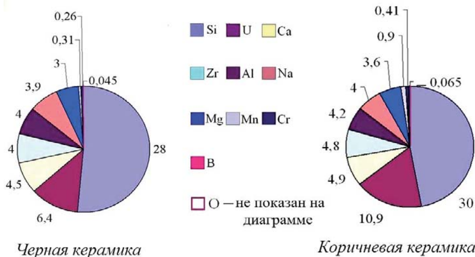
Рис. 15. Элементы (вес. %), входящие в состав различных модификаций ЛТСМ (образцы отобраны в ПРК)
