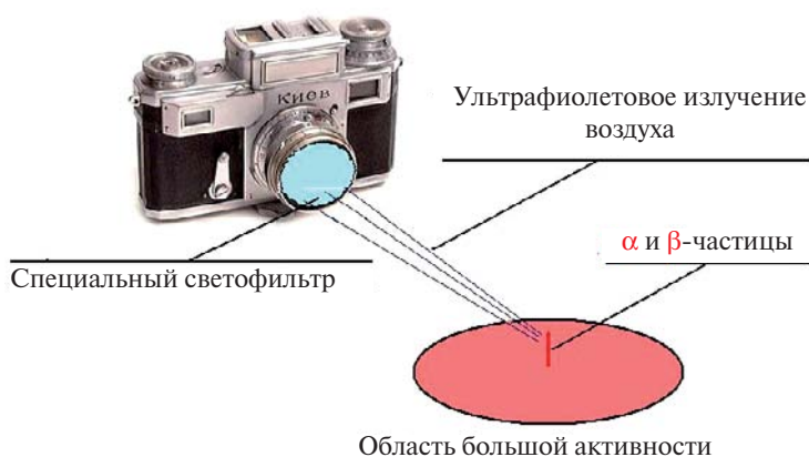
Рис. 7. Схема обнаружения областей с большой активностью с помощью фотографирования в ультрафиолетовом излучении
