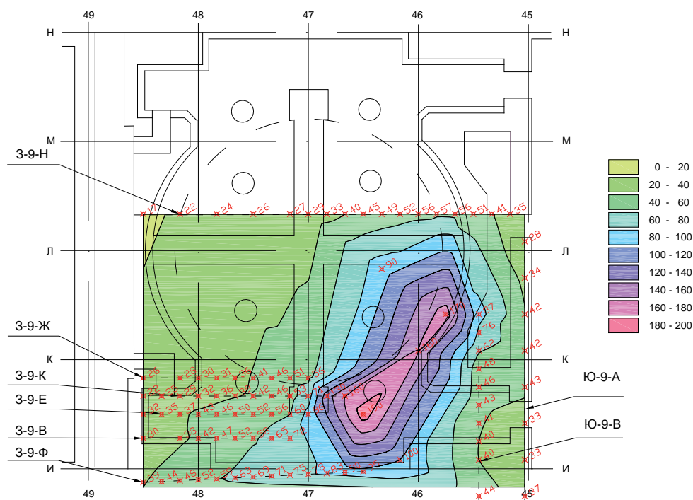
Рис. 13. Распределение температуры в подреакторной плите в ноябре 1988 г. (отм. 9.1 м)
