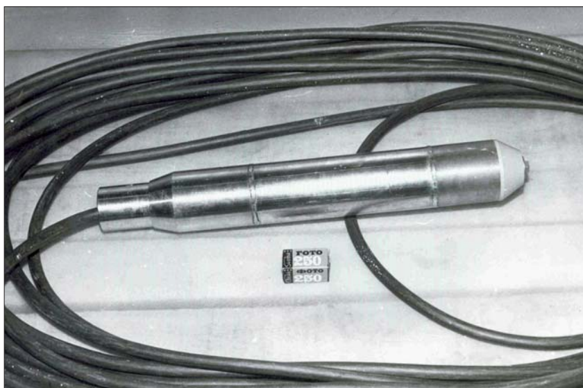
Рис. 2. Внешний вид прибора для измерений дозовых полей с помощью камеры «Сплав»
