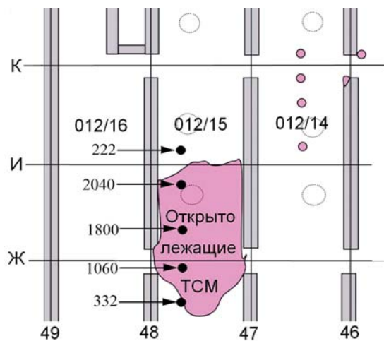
Рис. 28. Схема помещений ББ-2 и места расположения скоплений ЛТСМ. Приведены некоторые результаты измерений МЭД (Р/час), выполненные в январе 1989 г.
