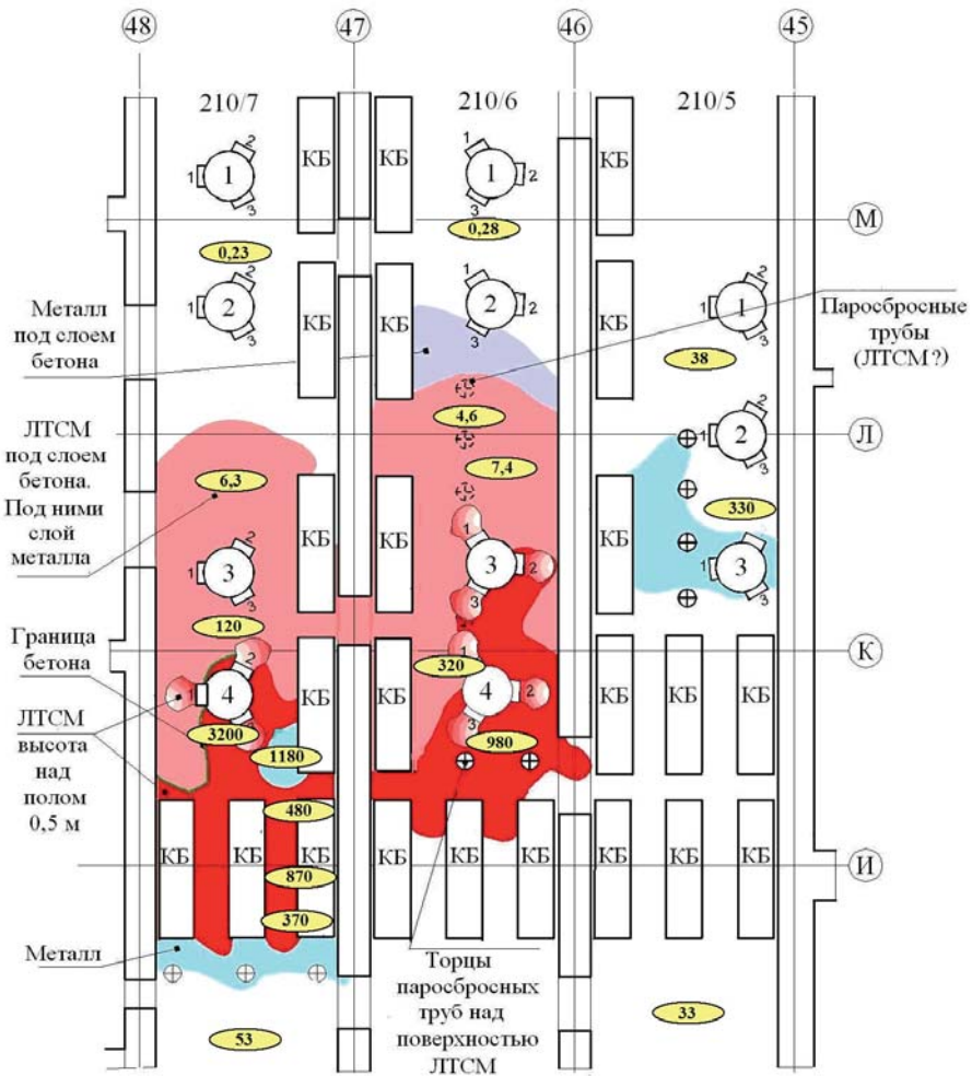
Рис. 25. ЛТСМ и металл в парораспределительном коридоре. Пом. 210/7 – «большой вертикальный поток», 210/6 – «малый вертикальный поток». Приведены некоторые результаты измерений МЭД (в желтых овалах, Р/час), выполненные в 2001 г.
