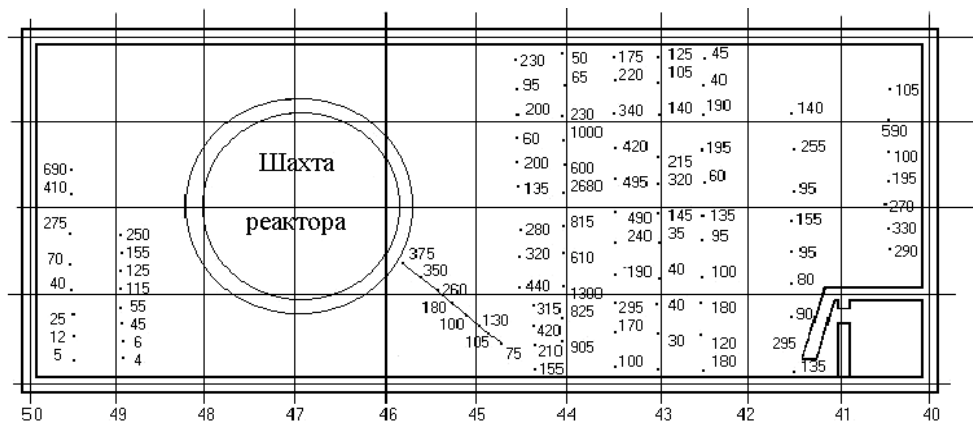
Рис. 4. Измерения величин мощностей экспозиционной дозы (Р/ч) в ЦЗ, проведенные в 1988 г. с помощью континуальных дозиметрических шнуров
